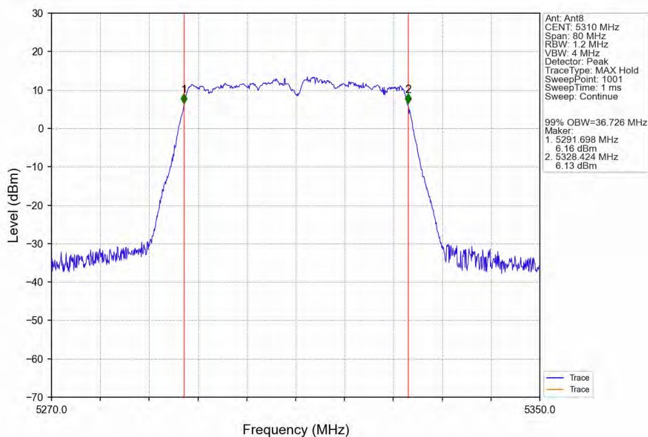
802.11n(HT40)_HCH_5310MHz_Ant8_NTNV
