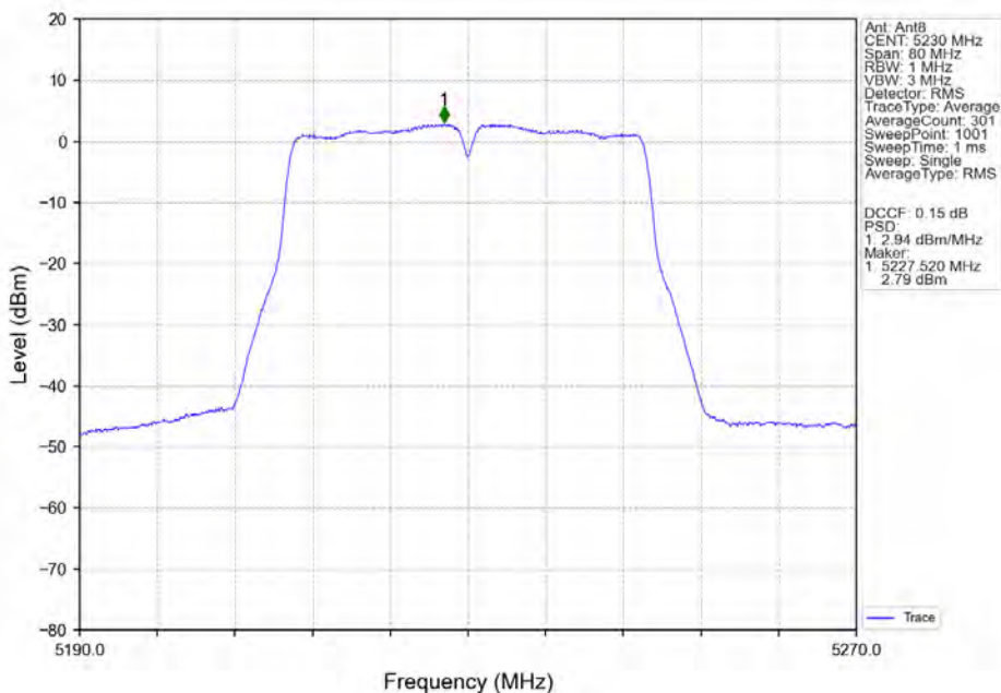
802.11n(HT40)_HCH_5230MHz_Ant8_NTNV
