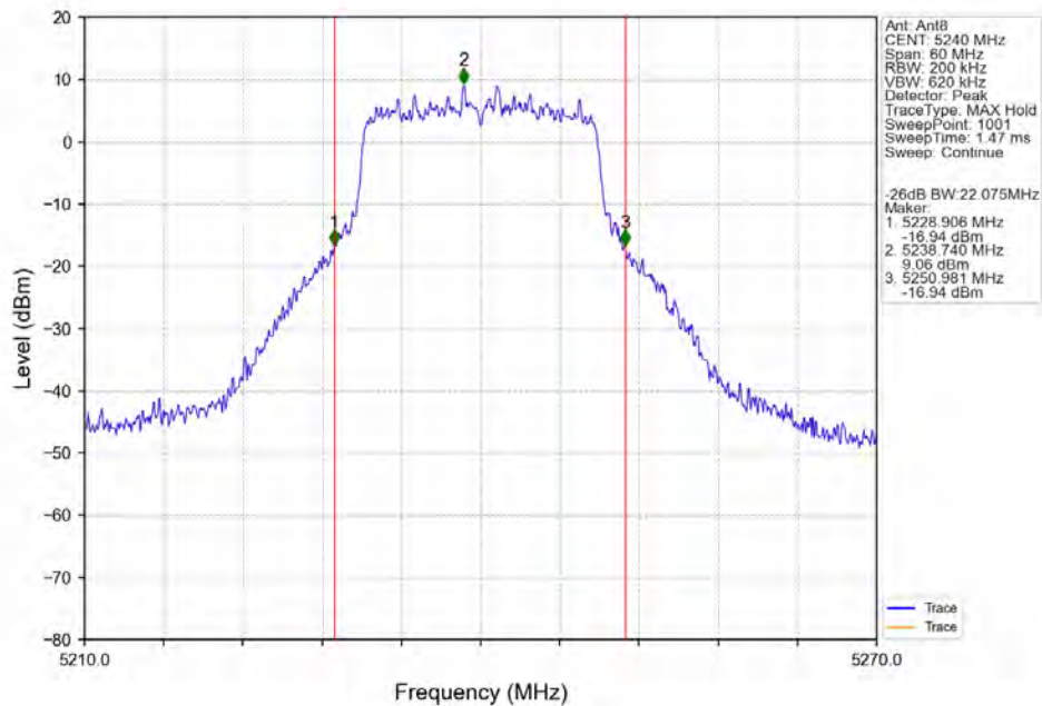
802.11n(HT20) HCH 5240MHz Ant8 NTN
