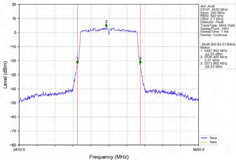
802.11ac(VHT80) LCH 5530MHz Ant8 NTN
