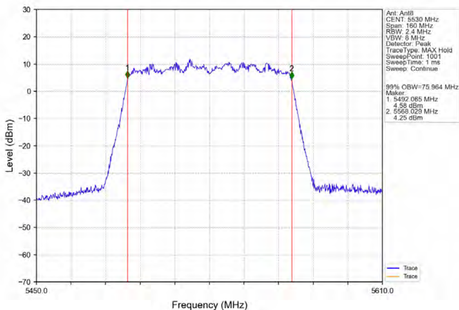
802.11ac(VHT80)_LCH_5530MHz_Ant8_NTNV
