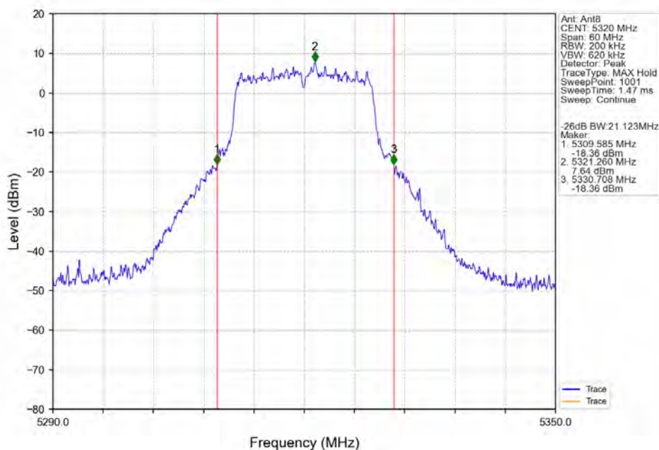
802.11a HCH 5320MHz Ant8 NTN
