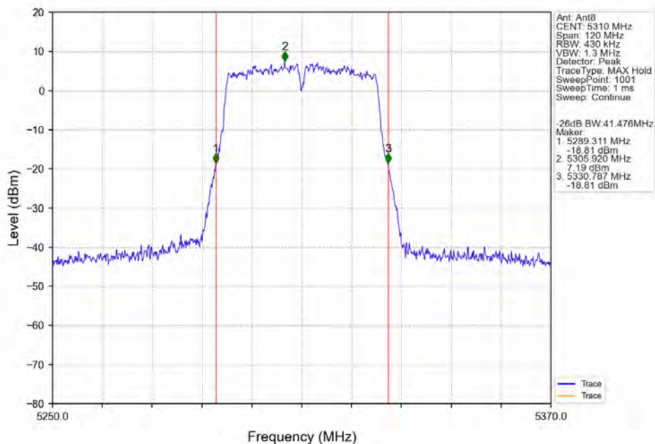
802.11n(HT40) HCH 5310MHz Ant8 NTNV
