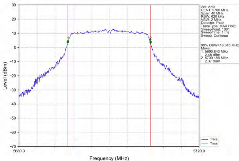
802.11ac(VHT20)_HCH_5700MHz_Ant8_NTNV
