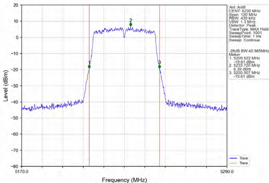
802.11ac(VHT40) HCH 5230MHz Ant8 NTN
