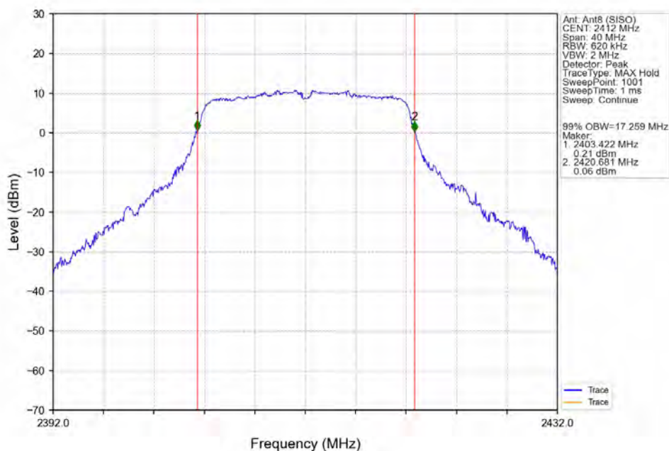
802.11g_LCH_2412MHz_Ant8 (SISO)_NTNV
