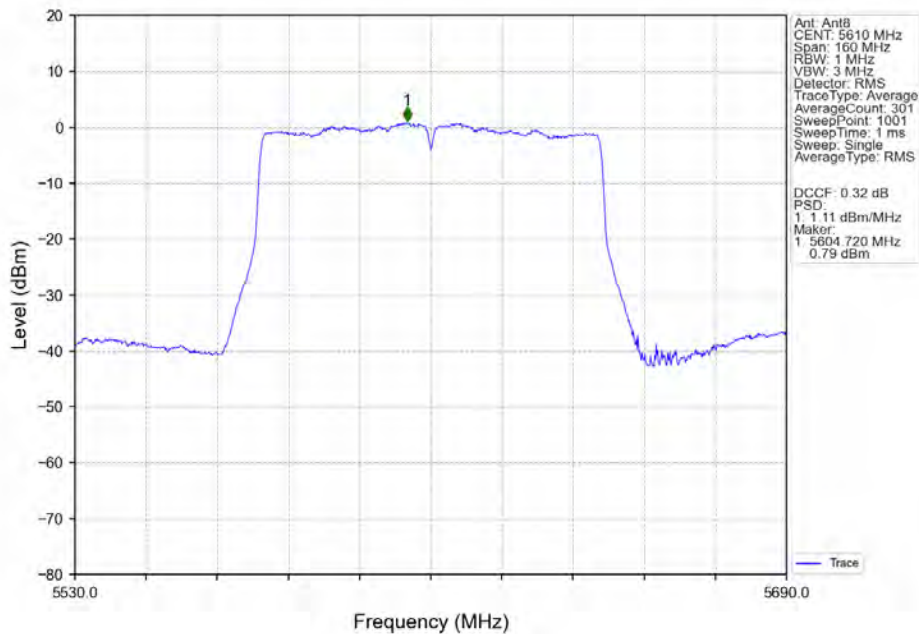
802.11ac(VHT80)_HCH_5610MHz_Ant8_NTNV
