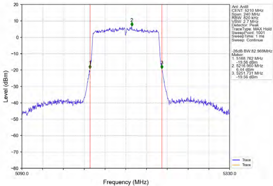
802.11ac(VHT80) MCH 5210MHz Ant8 NTN
