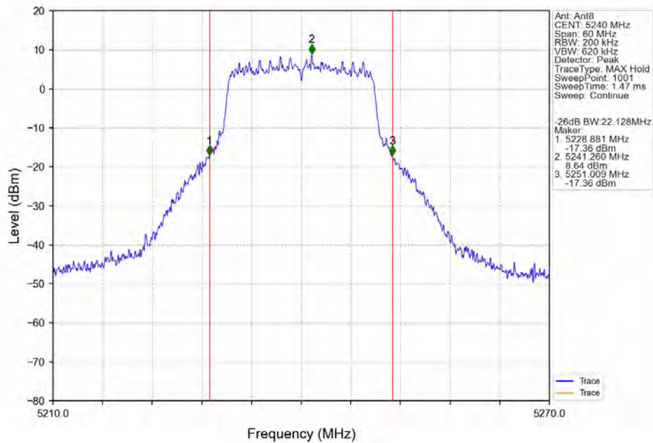
802.11ac(VHT20) HCH 5240MHz Ant8 NTN
