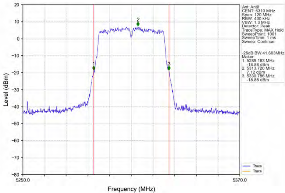
802.11ac(VHT40) HCH 5310MHz_Ant8_NTNV
