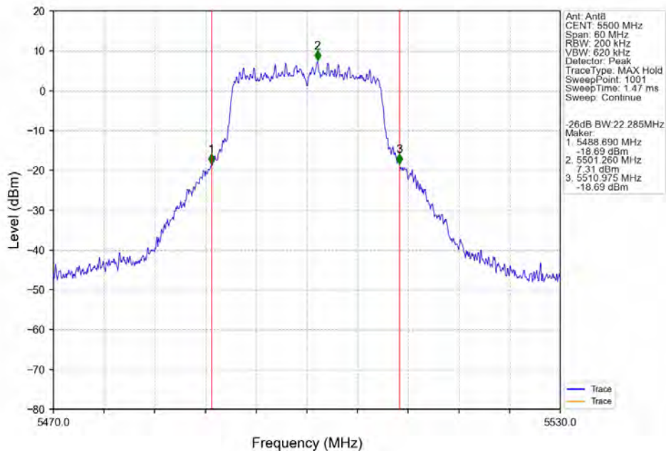
802.11n(HT20)_LCH_5500MHz_Ant8_NTNV
