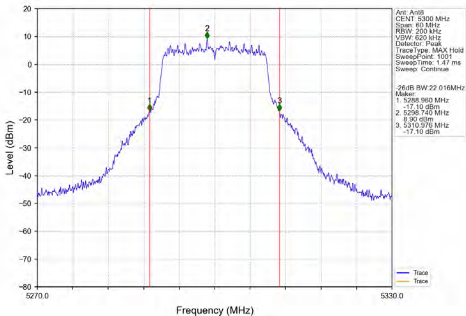
802.11ac(VHT20) MCH 5300MHz Ant8 NTN
