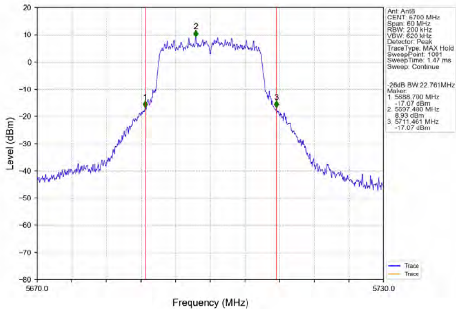
802.11ac(VHT20) HCH 5700MHz_Ant8_NTNV
