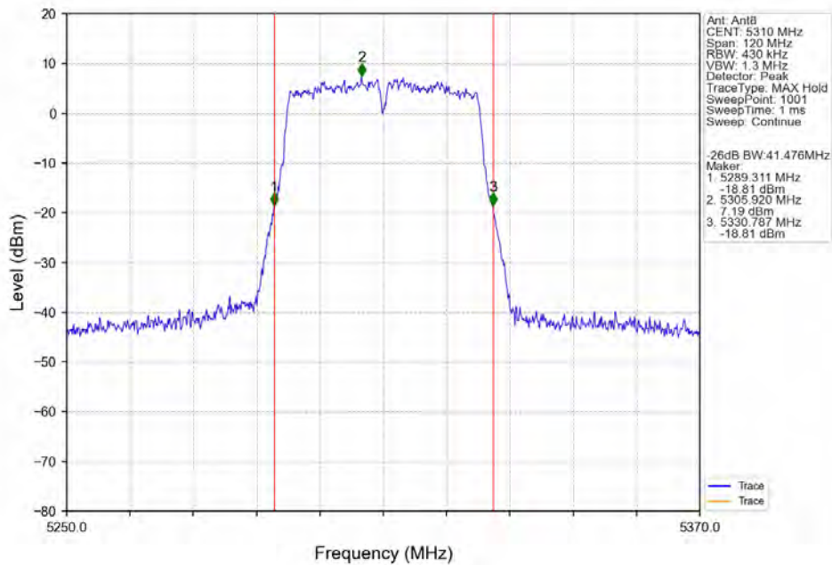
802.11n(HT40)_HCH_5310MHz_Ant8_NTNV
