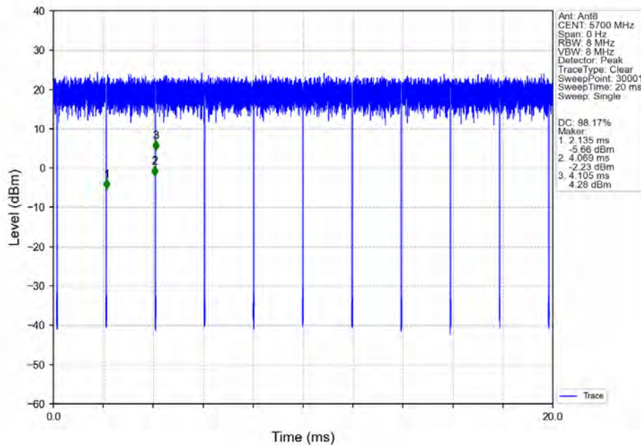
802.11ac(VHT20) HCH 5700MHz_Ant8_NTNV
