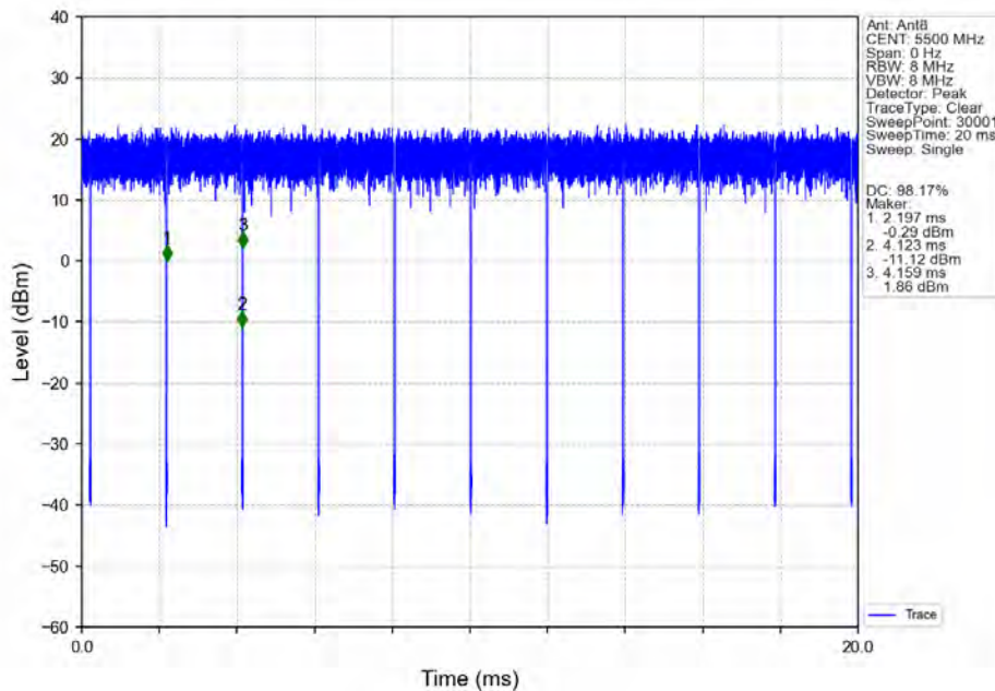
802.11n(HT20)_LCH_5500MHz_Ant8_NTNV
