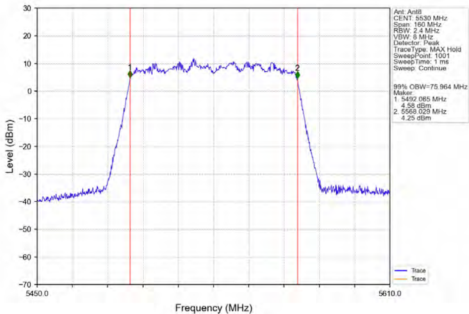
802.11ac(VHT80)_LCH_5530MHz_Ant8_NTNV
