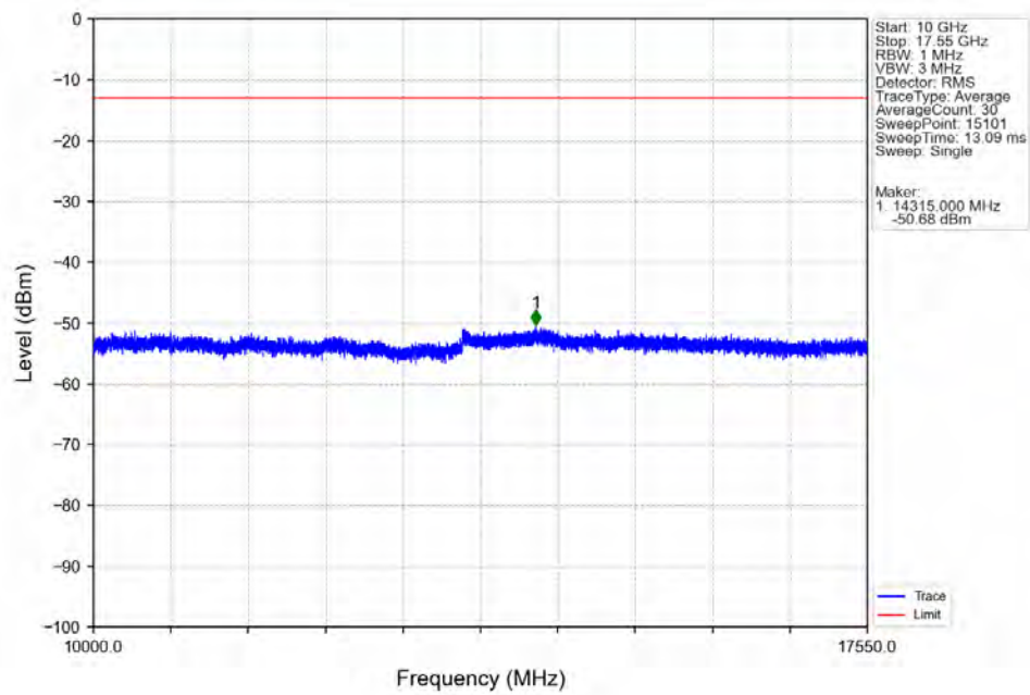
Band4 10MHz 64QAM HCH 1750MHz RB 1 0 NTNV
