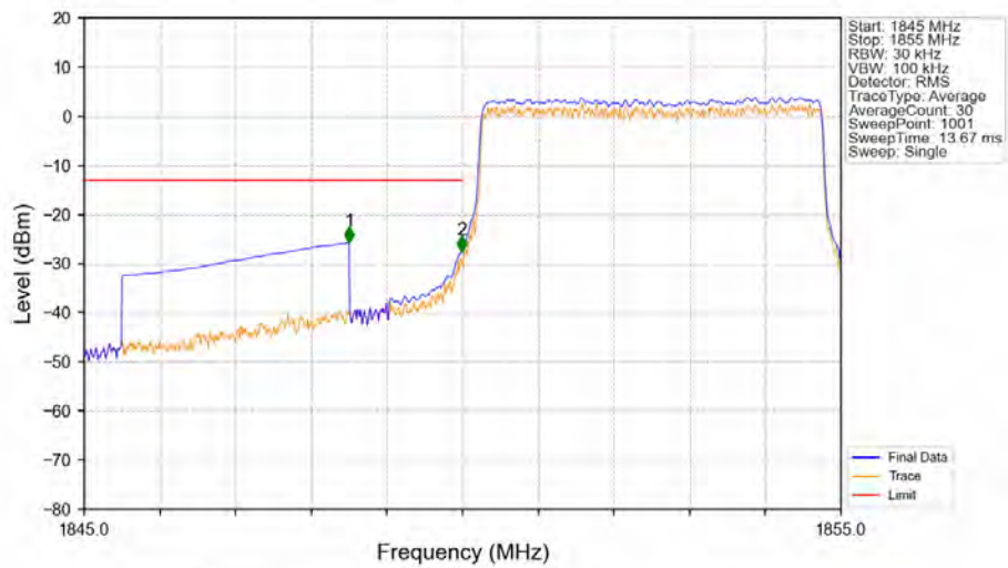
Band2 5MHz QPSK LCH 1852.5MHz RB 25 0 NTN
