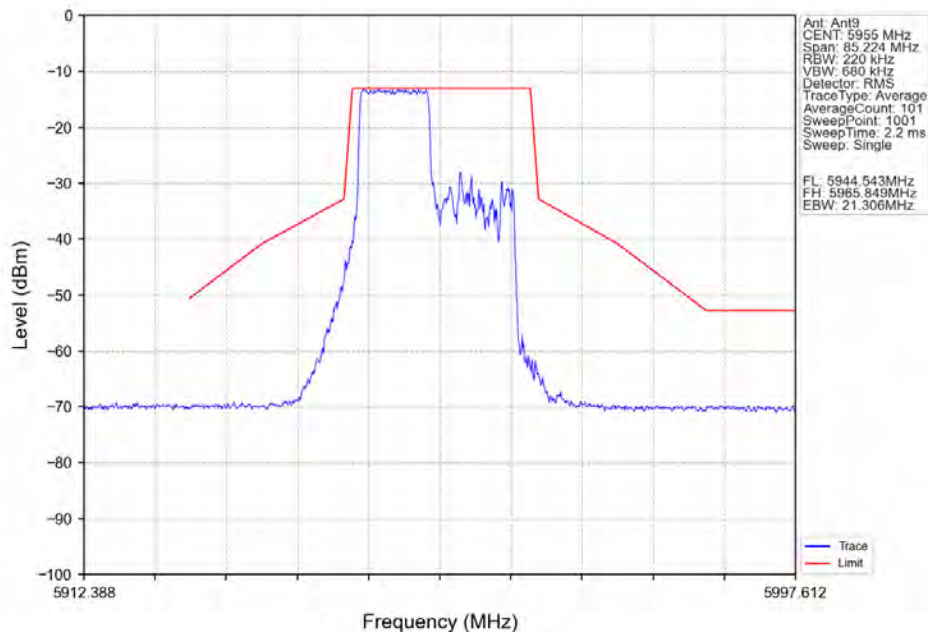
802.11ax(HEW20) LCH 5955MHz RU106 Left Ant9 NTVN
