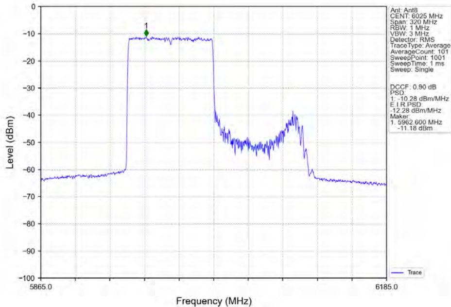
802.11ax(HEW160) LCH_6025MHz RU996 Left MIMO NTN
