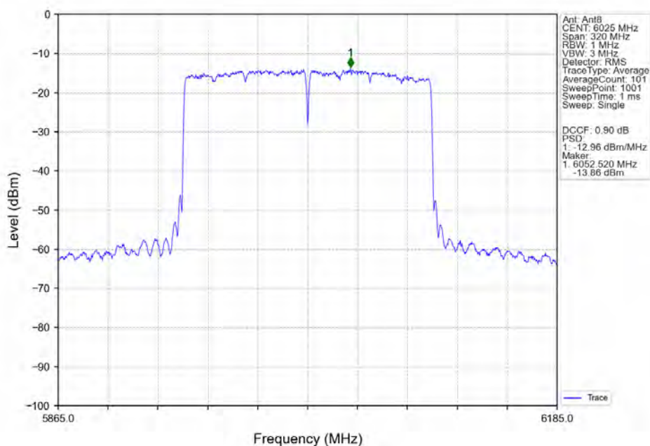
802.11ax(HEW160)_LCH_6025MHz_2xRU996_Left_Ant8_NTNV
