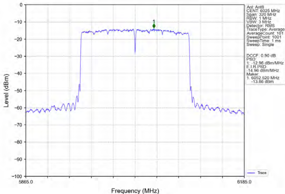
802.11ax(HEW160)_LCH_6025MHz_2xRU996_Left_Ant8_NTNV
