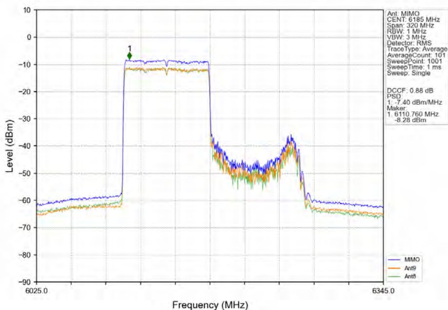
802.11ax(HEW160) MCH_6185MHz RU996 Left MIMO NTN
