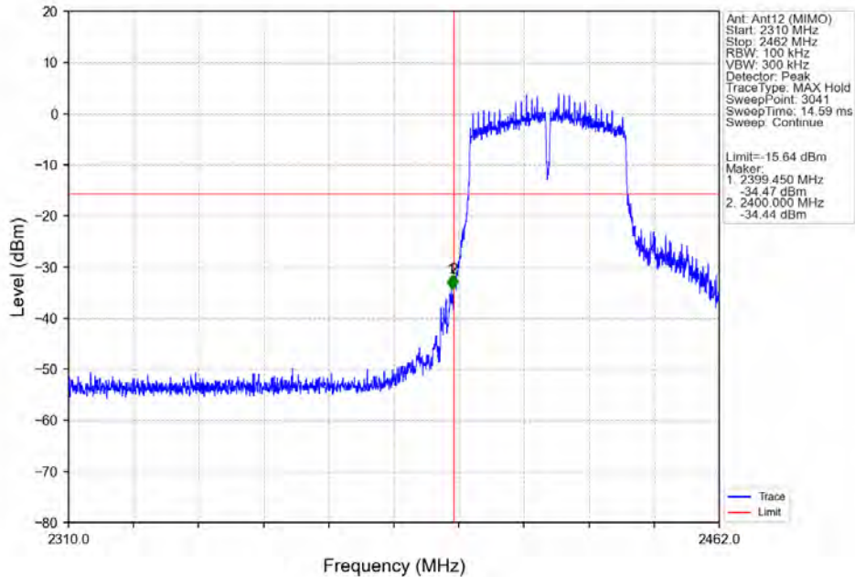
802.11n(HT40)_LCH_2422MHz_Ant12 (MIMO)_NTNV
