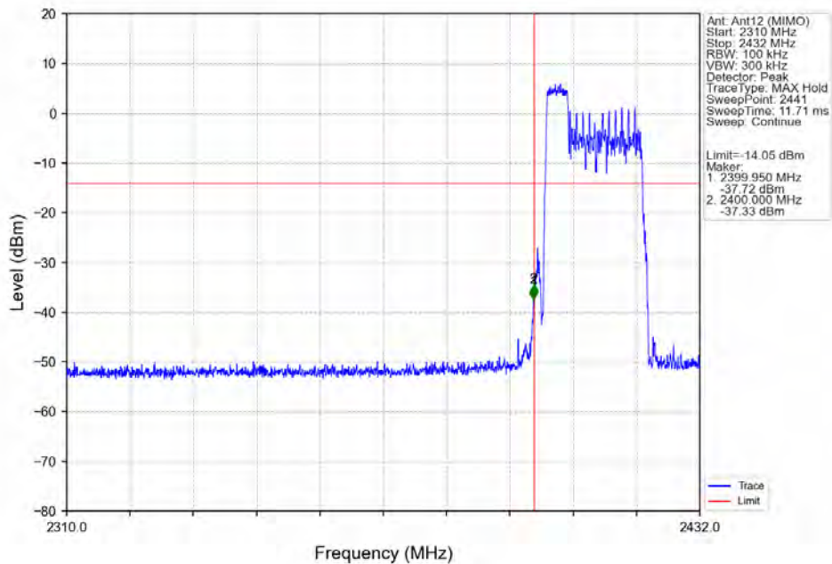
802.11ax(HEW20)_LCH_2412MHz_RU52_Left_Ant12 (MIMO)_NTNV
