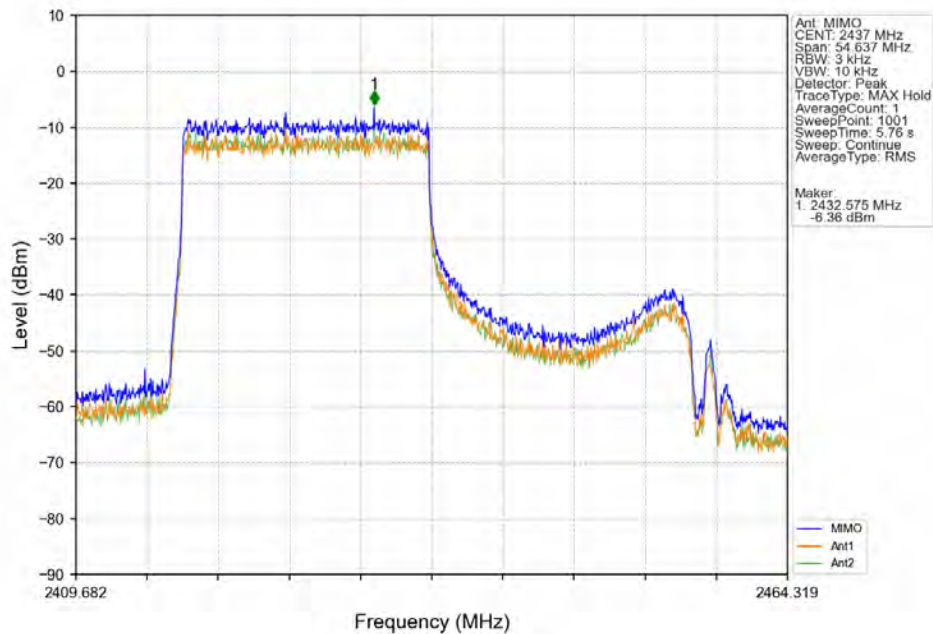
802.11ax(HEW40)_MCH_2437MHz_RU484_Left_Ant7 (MIMO)_NTNV
