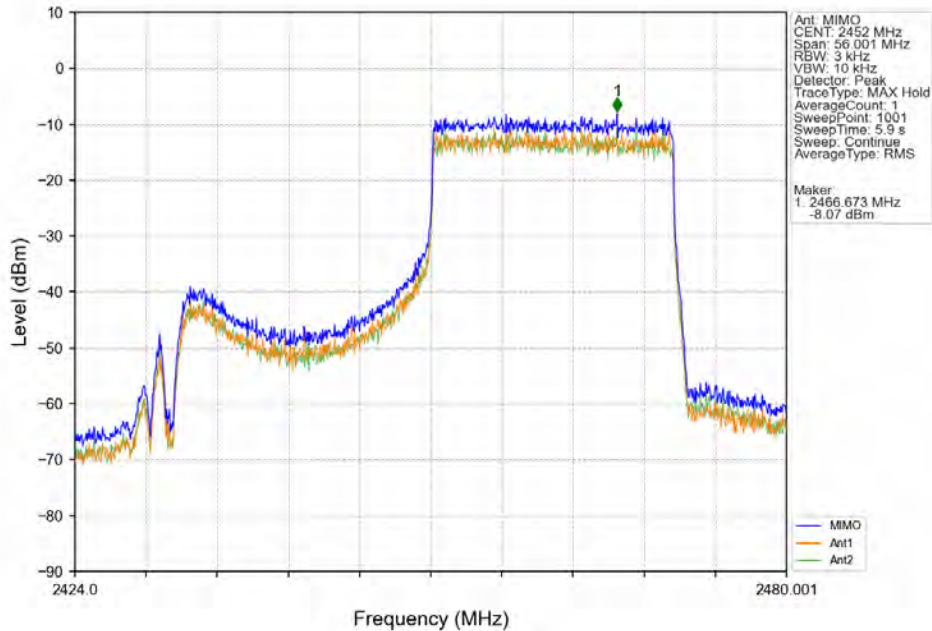
802.11ax(HEW40)_HCH_2452MHz_RU484_Left_Ant7 (MIMO)_NTNV
