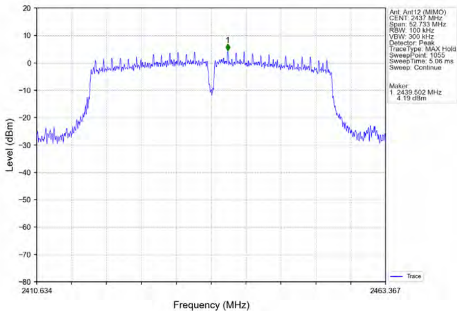
802.11ac(VHT40)_MCH_2437MHz_Ant12 (MIMO)_NTNV
