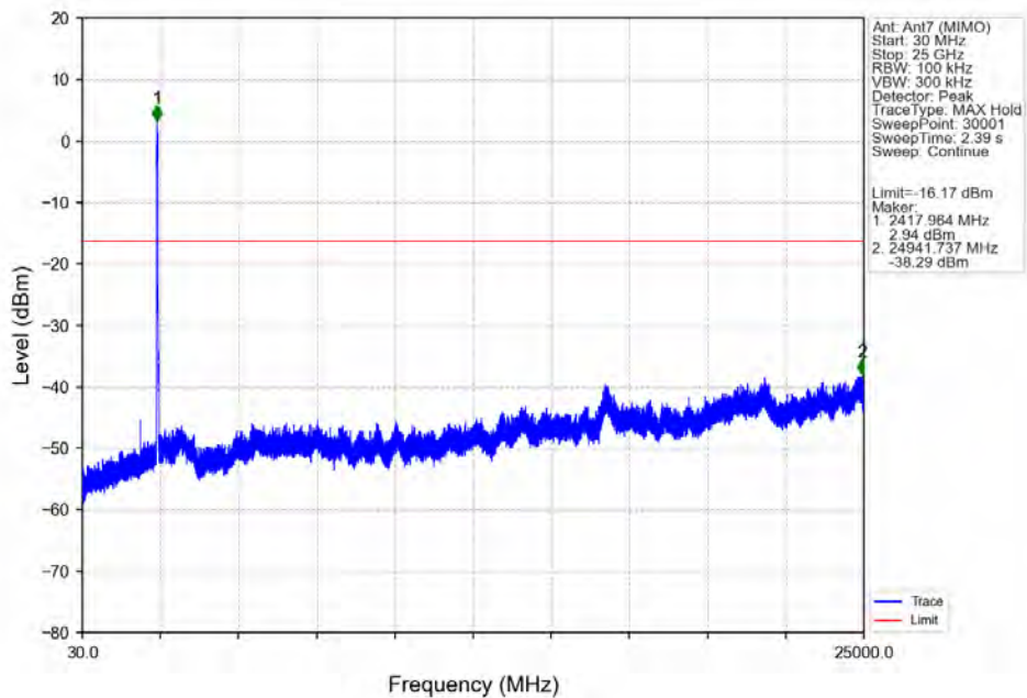
802.11n(HT40)_LCH_2422MHz_Ant7 (MIMO)_NTNV
