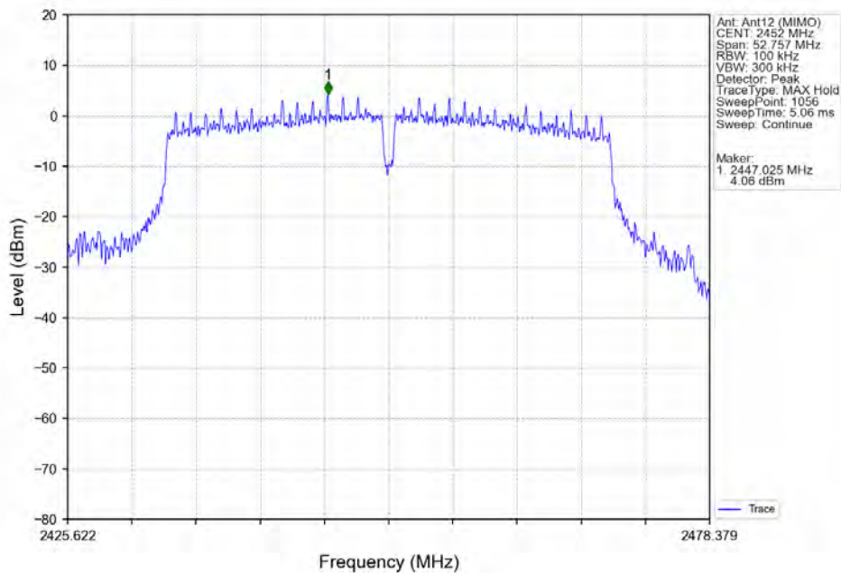
802.11n(HT40)_HCH_2452MHz_Ant12 (MIMO)_NTNV
