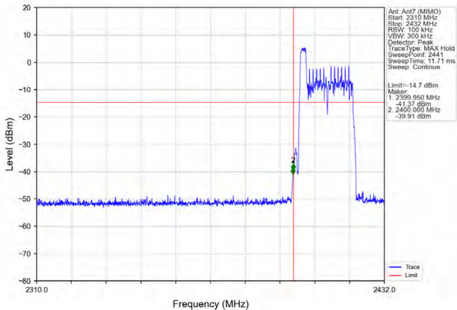
802.11ax(HEW20)_LCH_2412MHz_RU26_Left_Ant7 (MIMO)_NTNV
