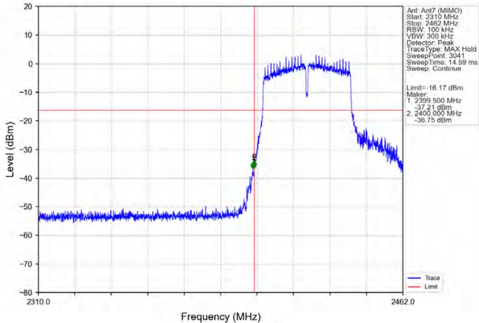
802.11n(HT40)_LCH_2422MHz_Ant7 (MIMO)_NTNV
