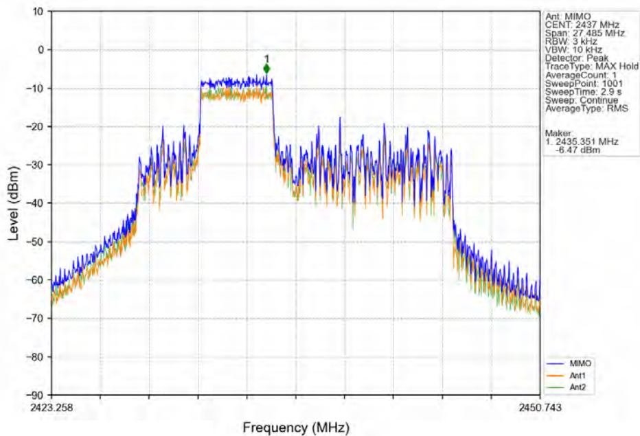
802.11ax(HEW20)_MCH_2437MHz_RU52_Mid_MIMO_NTNV
