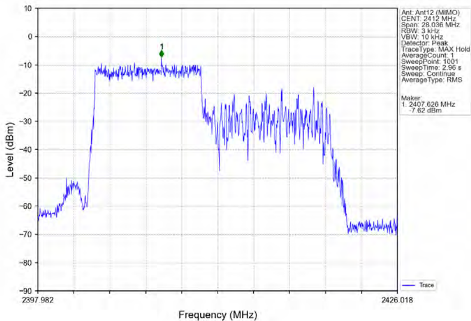
802.11ax(HEW20)_LCH_2412MHz_RU106_Left_Ant12 (MIMO)_NTNV
