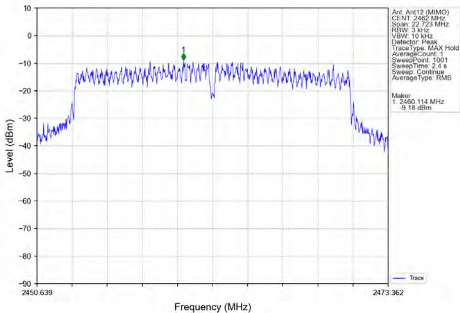
802.11n(HT20)_HCH_2462MHz_Ant12 (MIMO)_NTNV
