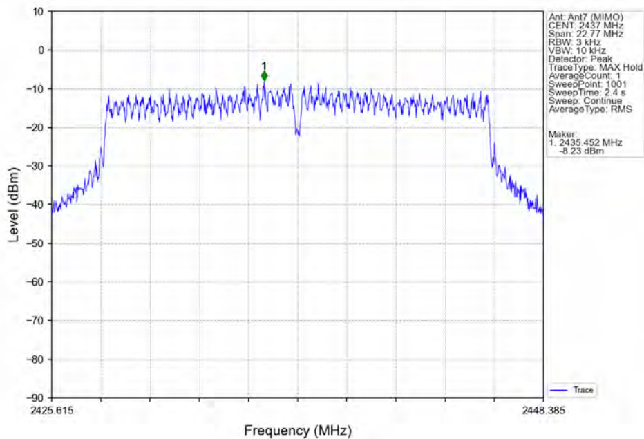
802.11n(HT20)_MCH_2437MHz_Ant7 (MIMO)_NTNV
