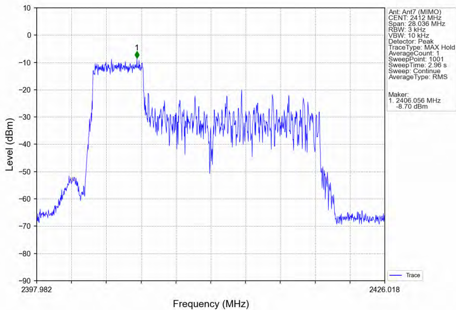
802.11ax(HEW20)_LCH_2412MHz_RU52_Left_Ant7 (MIMO)_NTNV
