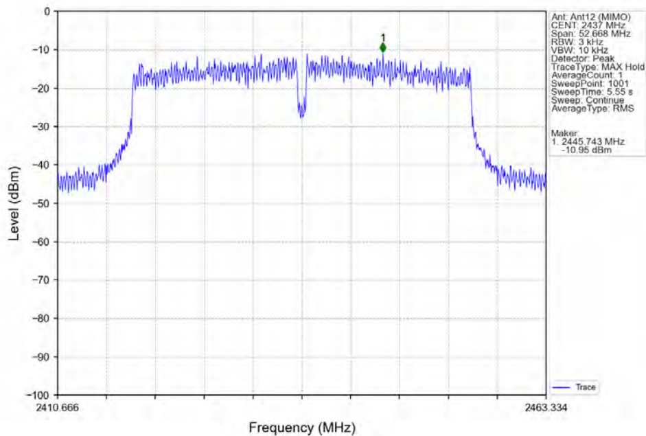
802.11n(HT40)_MCH_2437MHz_Ant12 (MIMO)_NTNV
