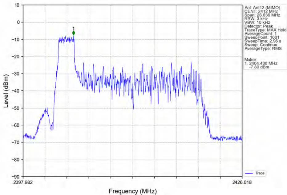
802.11ax(HEW20)_LCH_2412MHz_RU26_Left_Ant12 (MIMO)_NTNV
