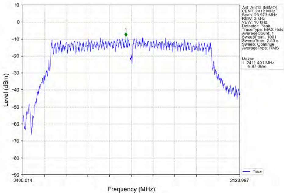
802.11n(HT20)_LCH_2412MHz_Ant12 (MIMO)_NTNV
