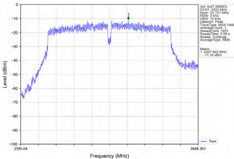
802.11n(HT40)_LCH_2422MHz_Ant7 (MIMO)_NTNV
