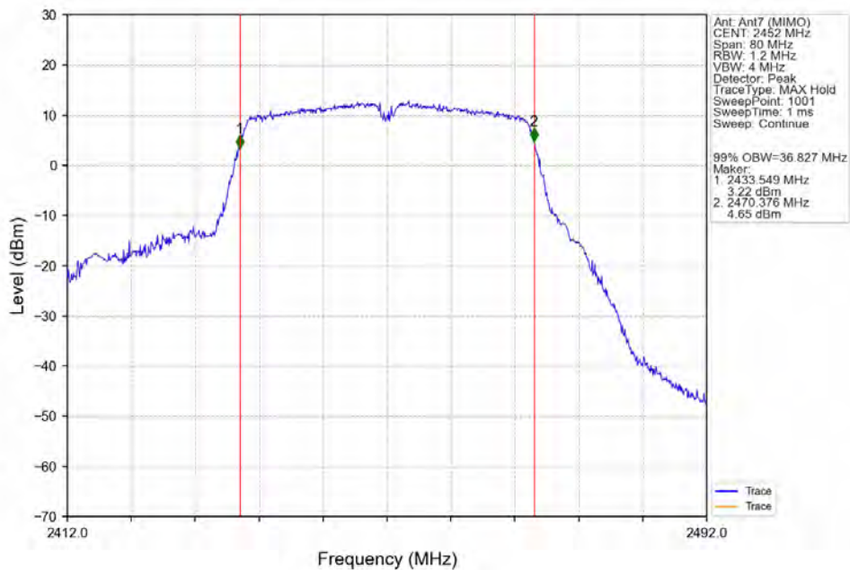
802.11n(HT40)_HCH_2452MHz_Ant7 (MIMO)_NTNV
