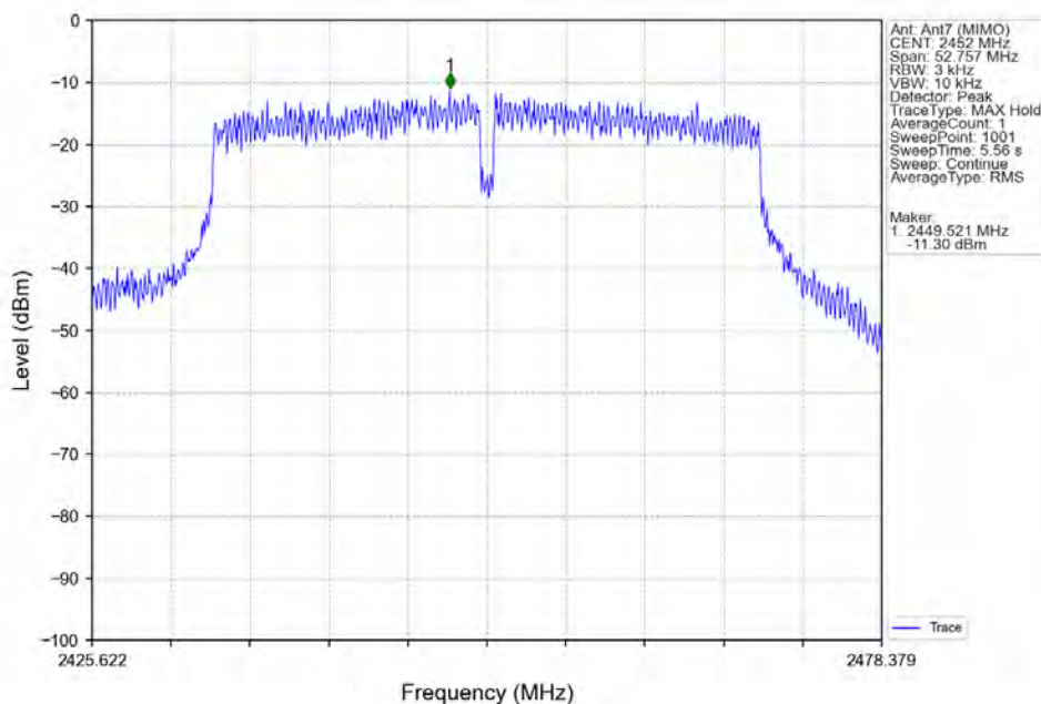
802.11n(HT40)_HCH_2452MHz_Ant7 (MIMO)_NTNV
