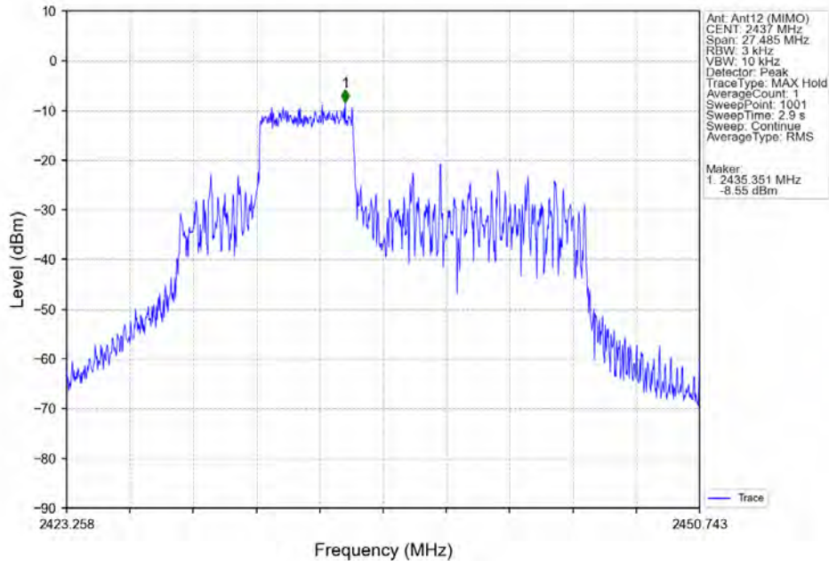
802.11ax(HEW20)_MCH_2437MHz_RU52_Mid_MIMO_NTNV
