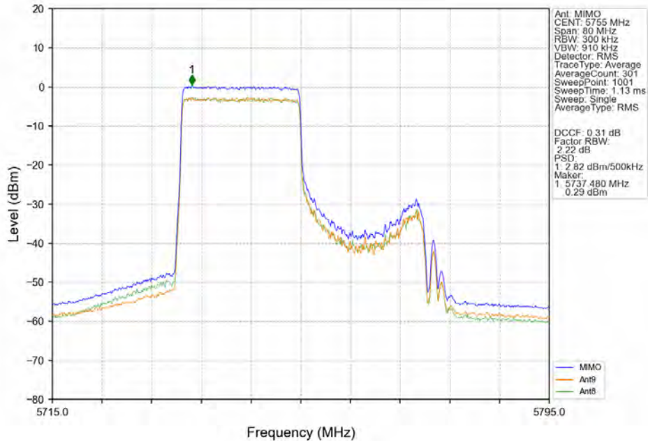
802.11ax(HEW40)_LCH_5755MHz_RU484_Left_Ant9_NTNV
