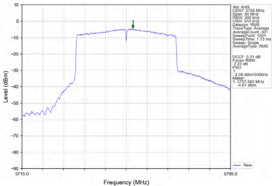
802.11ax(HEW40)_LCH_5755MHz_RU484_Left_Ant9_NTNV
