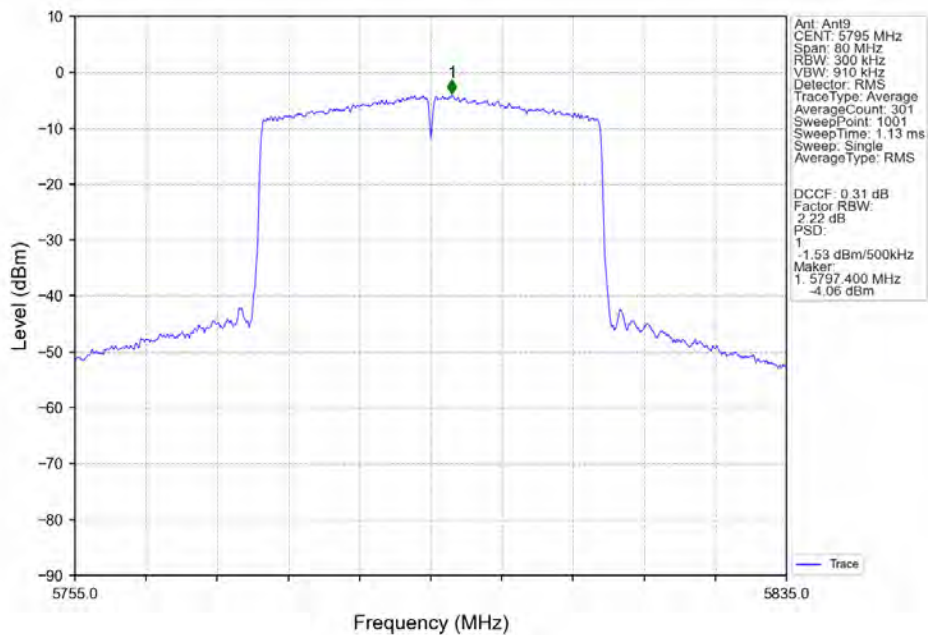
802.11ax(HEW40)_HCH_5795MHz_RU484_Left_Ant9_NTNV
