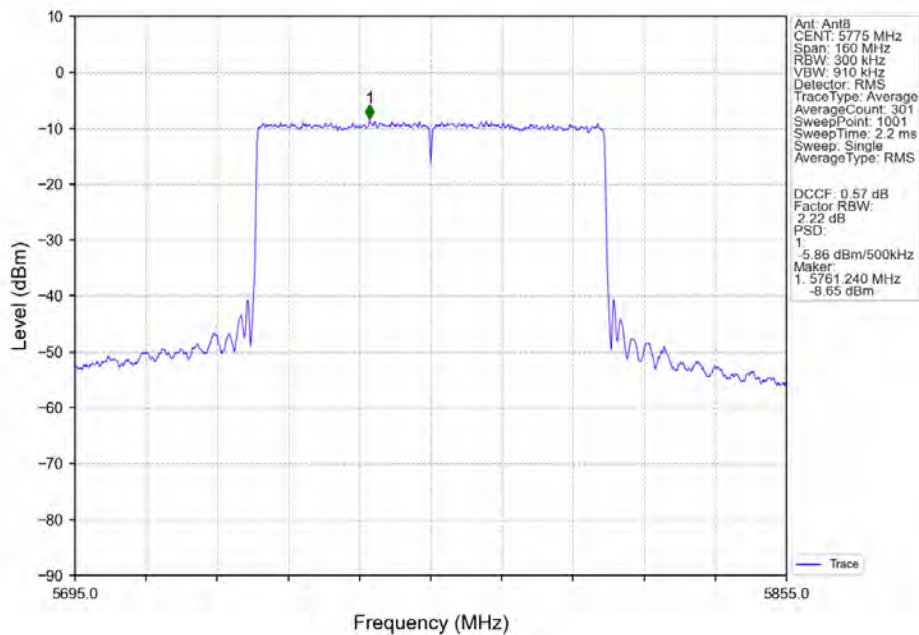
802.11ax(HEW80)_MCH_5775MHz_RU996_Left_Ant8_NTNV
