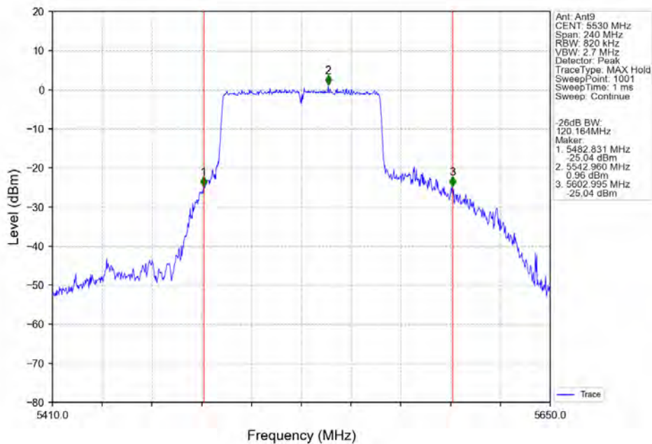
802.11ac(VHT80)_LCH_5530MHz_Ant9_NTNV
