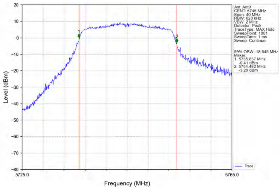
802.11n(HT20)_LCH_5745MHz_Ant9_NTNV
