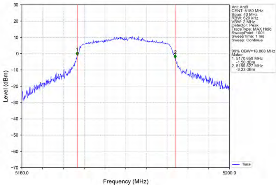
802.11ac(VHT20)_LCH_5180MHz_Ant9_NTNV
