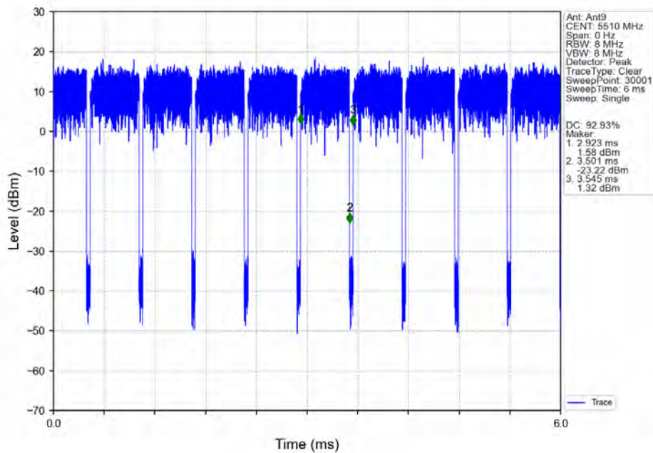
802.11ax(HEW40)_LCH_5510MHz_RU484_Left_Ant9_NTNV
