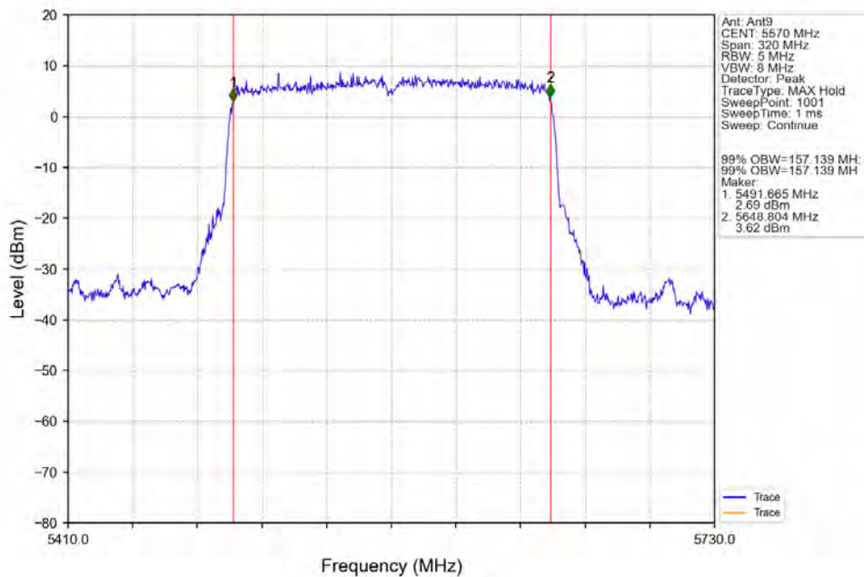
802.11ax(HEW160)_MCH_5570MHz_2xRU996_Left_Ant9_NTNV
