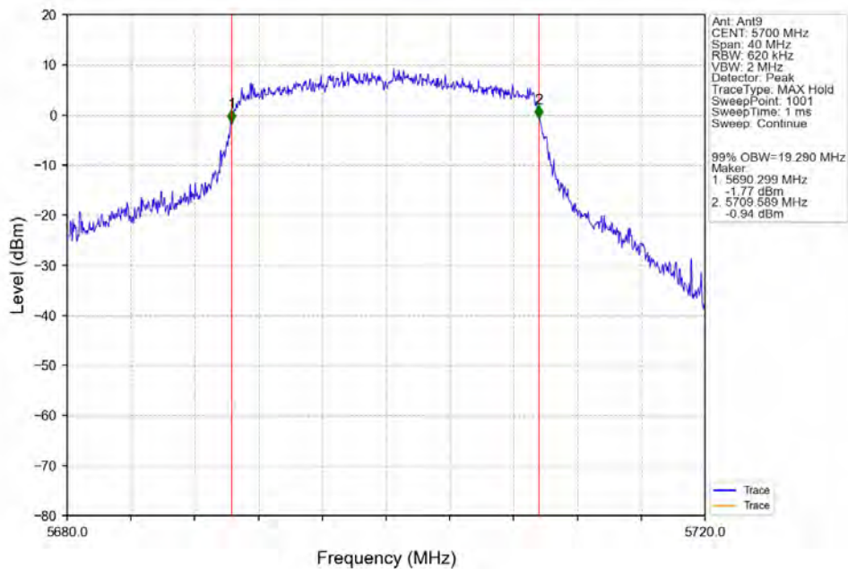
802.11ax(HEW20)_HCH_5700MHz_RU242_Left_Ant9_NTNV
