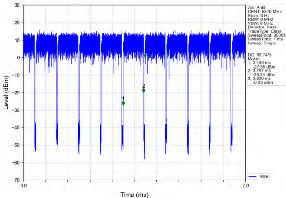
802.11n(HT40)_HCH_5310MHz_Ant9_NTNV
