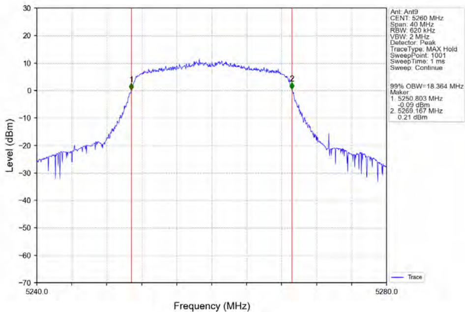
802.11n(HT20)_LCH_5260MHz_Ant9_NTNV
