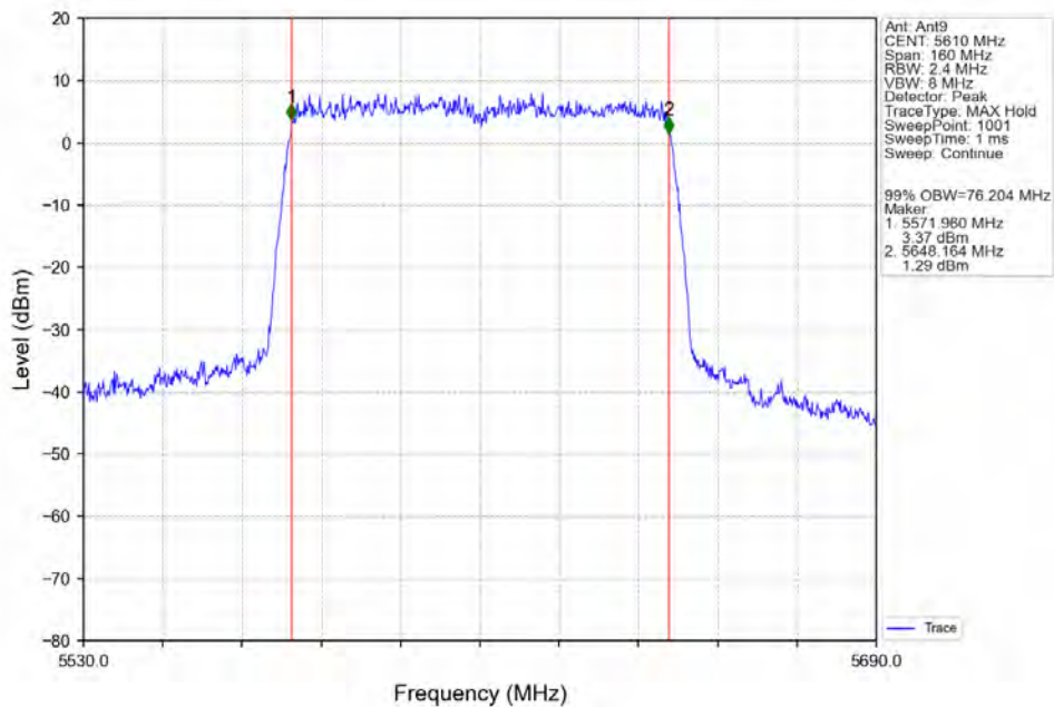
802.11ac(VHT80)_HCH_5610MHz_Ant9_NTNV
