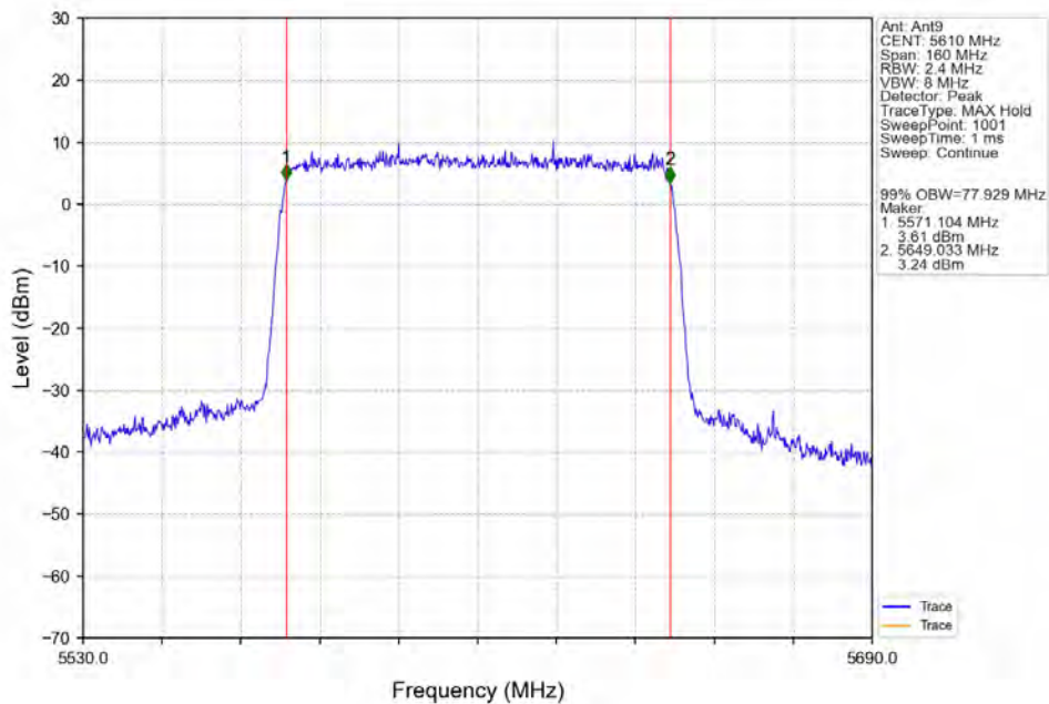
802.11ax(HEW80)_HCH_5610MHz_RU996_Left_Ant9_NTNV
