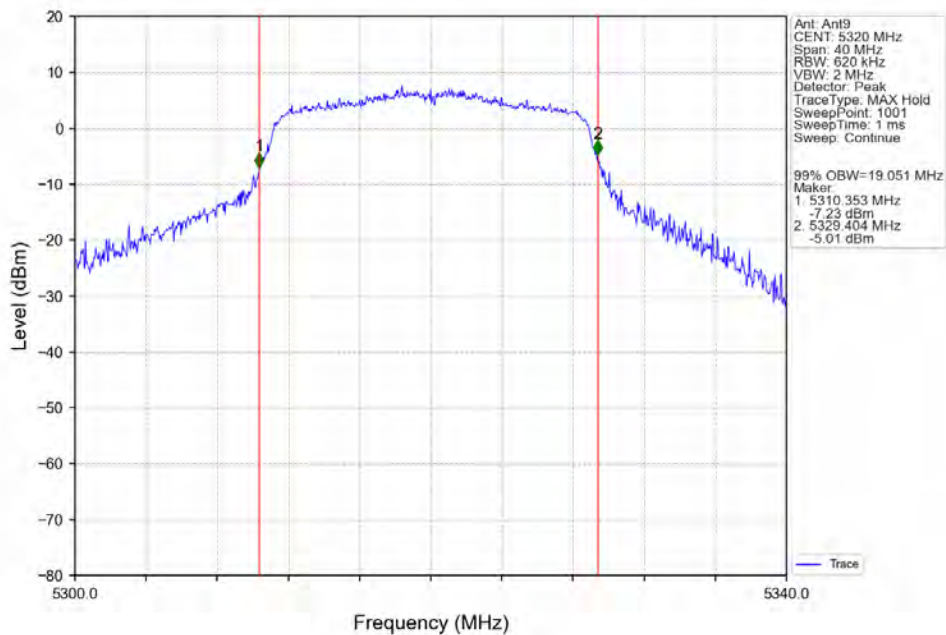
802.11n(HT20)_HCH_5320MHz_Ant9_NTNV
