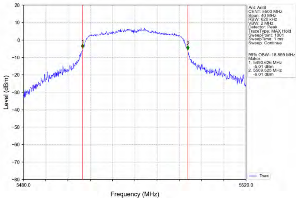
802.11ac(VHT20)_LCH_5500MHz_Ant9_NTNV
