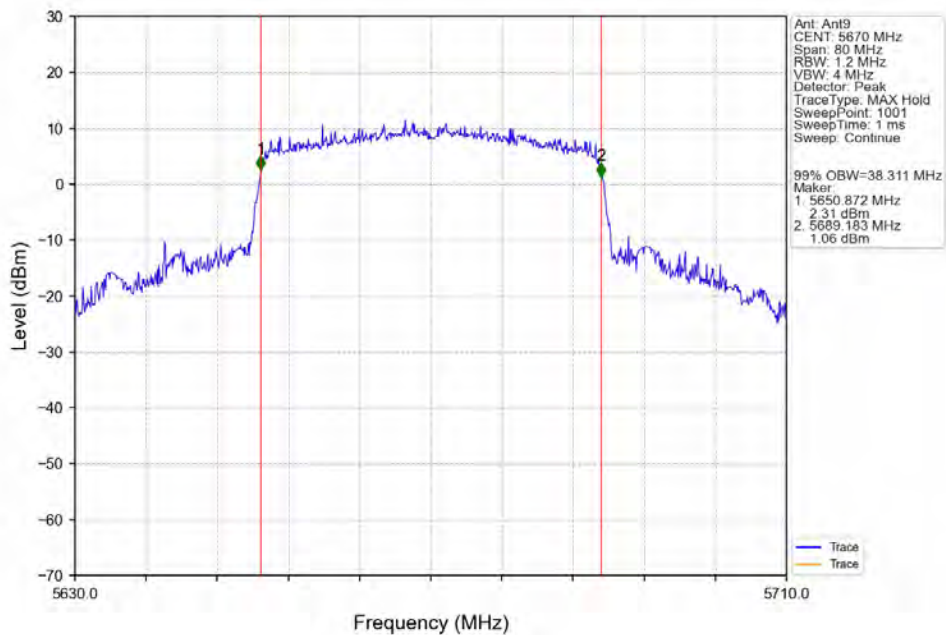
802.11ax(HEW40)_HCH_5670MHz_RU484_Left_Ant9_NTNV
