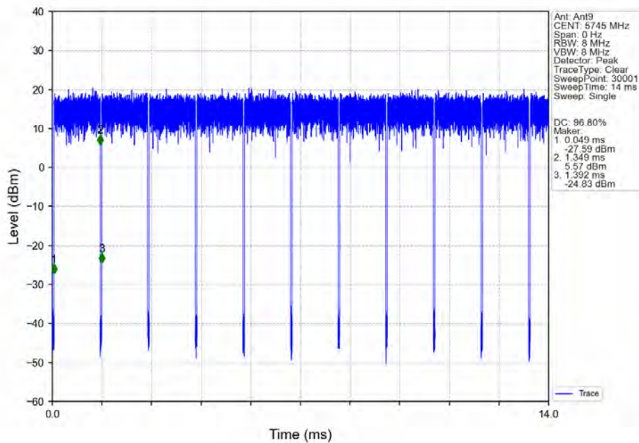
802.11n(HT20)_LCH_5745MHz_Ant9_NTNV
