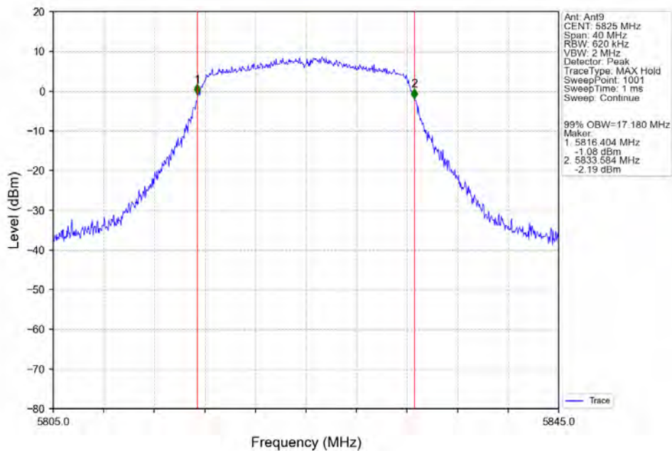
802.11a_HCH_5825MHz_Ant9_NTNV
