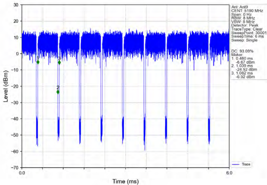
802.11ax(HEW40)_LCH_5190MHz_RU484_Left_Ant9_NTNV
