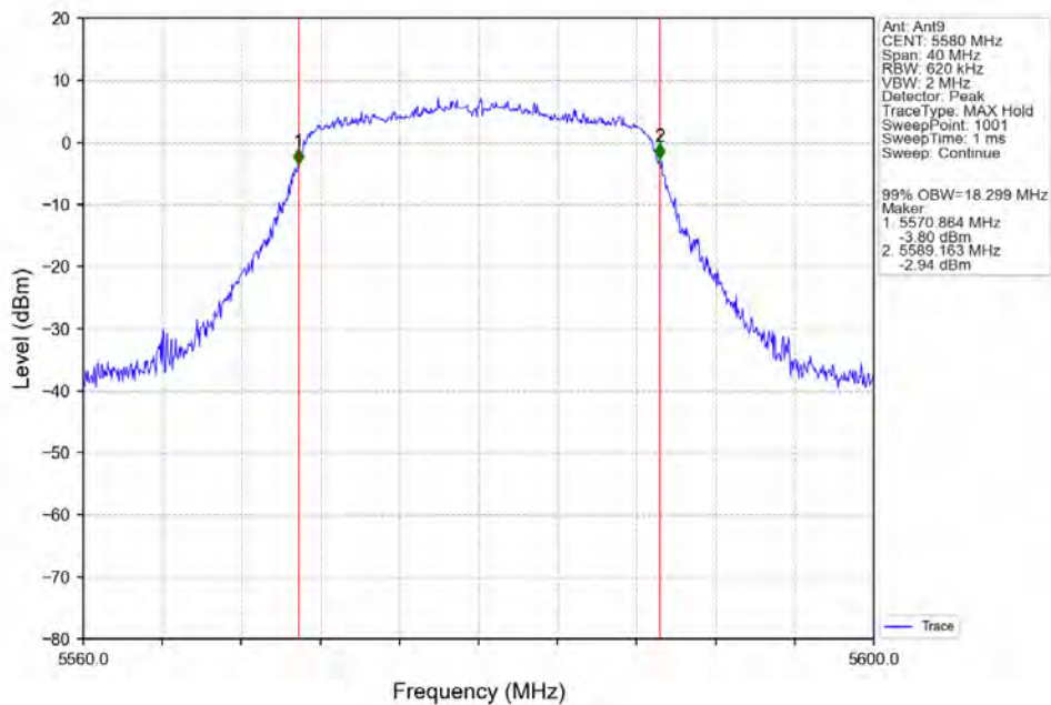
802.11n(HT20)_MCH_5580MHz_Ant9_NTNV
