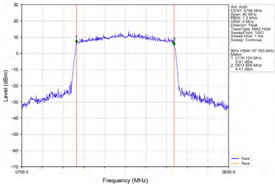
802.11ax(HEW40)_HCH_5795MHz_RU484_Left_Ant9_NTNV
