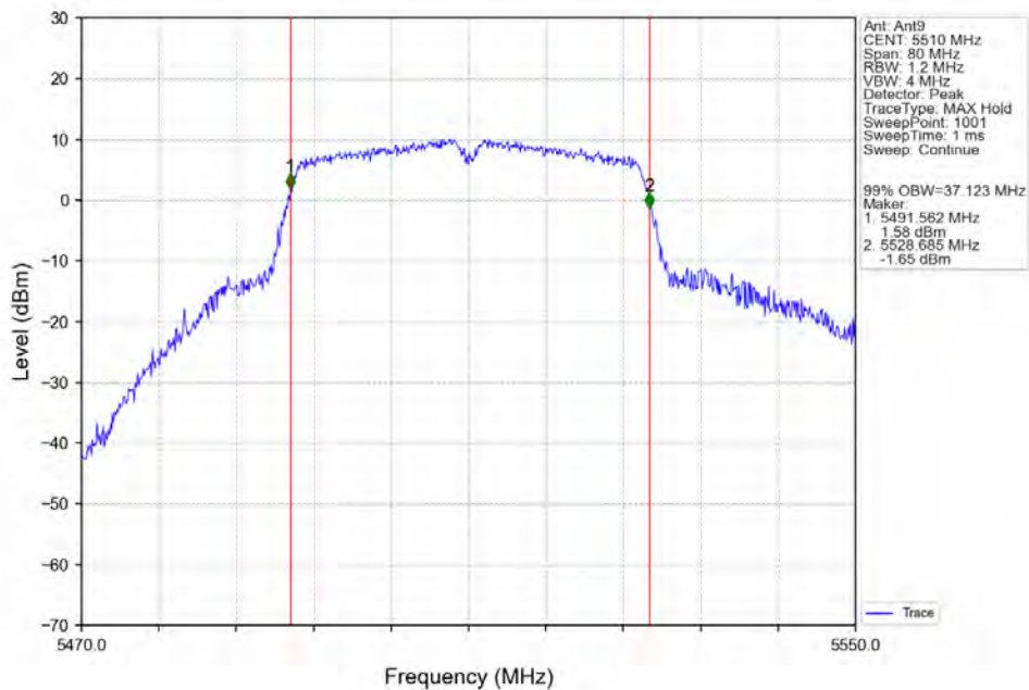
802.11ac(VHT40)_LCH_5510MHz_Ant9_NTNV
