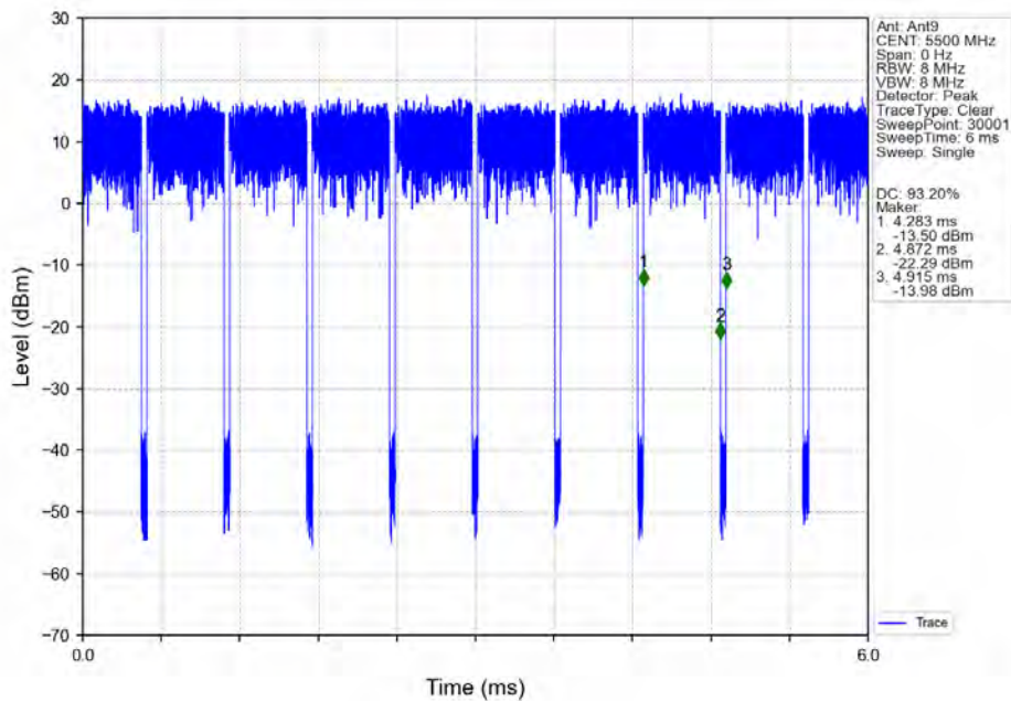
802.11ax(HEW20)_LCH_5500MHz_RU242_Left_Ant9_NTNV
