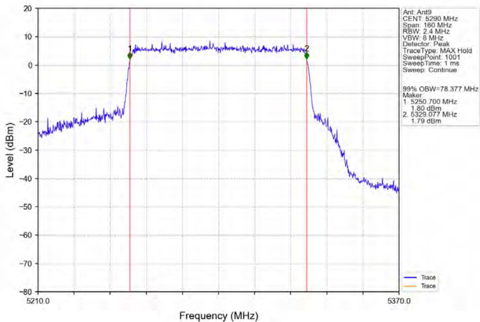
802.11ax(HEW80)_MCH_5290MHz_RU996_Left_Ant9_NTNV
