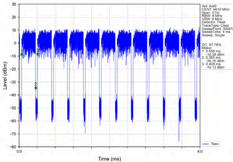
802.11ax(HEW80)_HCH_5610MHz_RU996_Left_Ant9_NTNV
