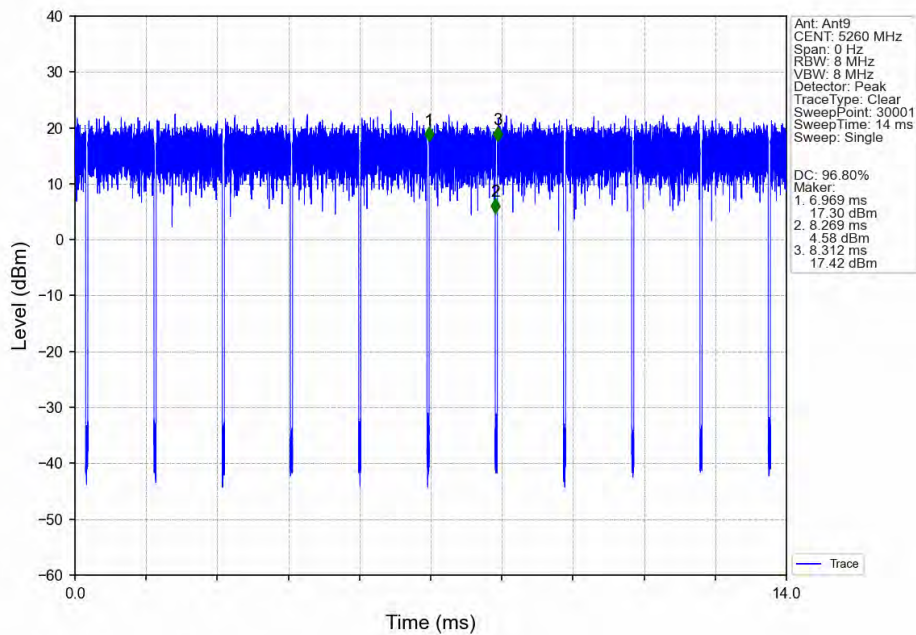
802.11n(HT20)_LCH_5260MHz_Ant9_NTNV
