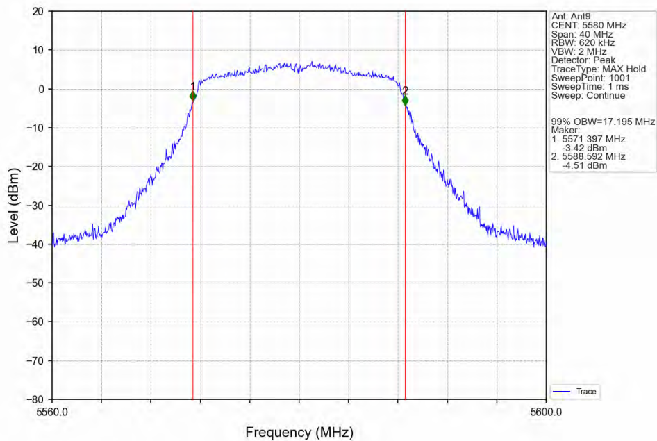
802.11a_MCH_5580MHz_Ant9_NTNV
