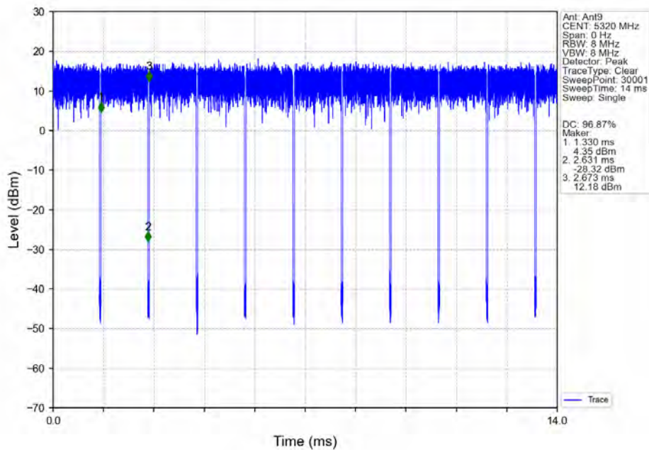
802.11n(HT20)_HCH_5320MHz_Ant9_NTNV
