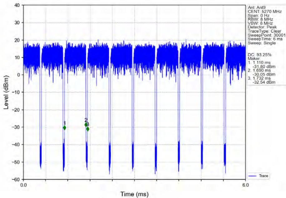
802.11ax(HEW40)_LCH_5270MHz_RU484_Left_Ant9_NTNV
