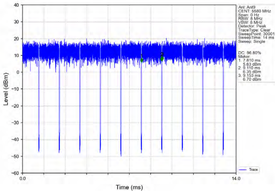
802.11n(HT20)_MCH_5580MHz_Ant9_NTNV
