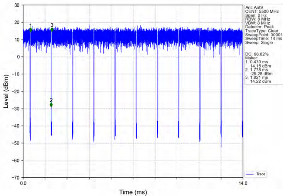
802.11ac(VHT20)_LCH_5500MHz_Ant9_NTNV
