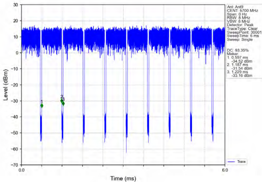
802.11ax(HEW20)_HCH_5700MHz_RU242_Left_Ant9_NTNV
