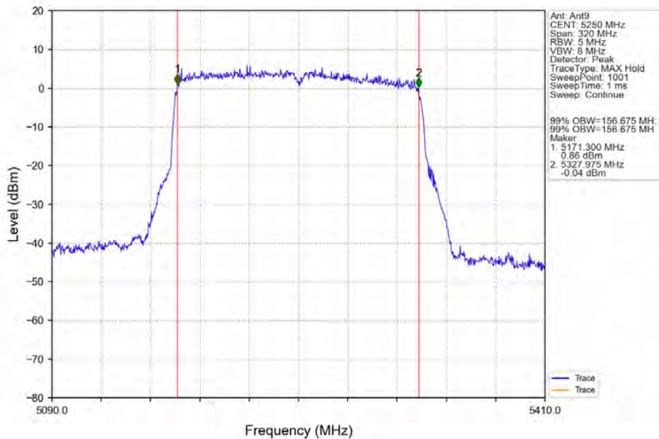
802.11ax(HEW160)_MCH_5250MHz_2xRU996_Left_Ant9_NTNV
