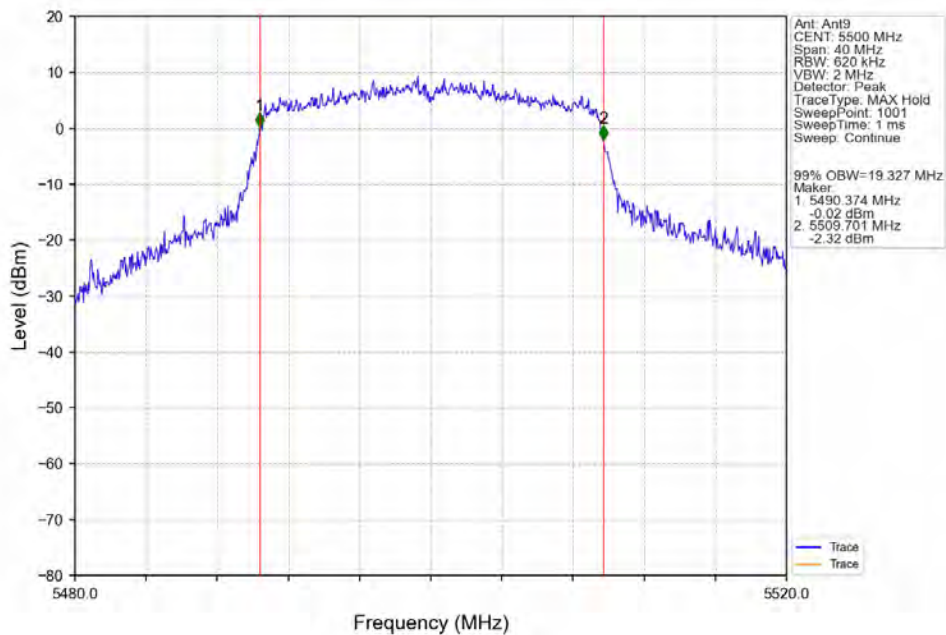
802.11ax(HEW20)_LCH_5500MHz_RU242_Left_Ant9_NTNV
