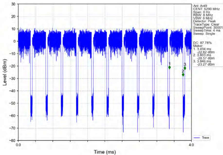
802.11ax(HEW80)_MCH_5290MHz_RU996_Left_Ant9_NTNV
