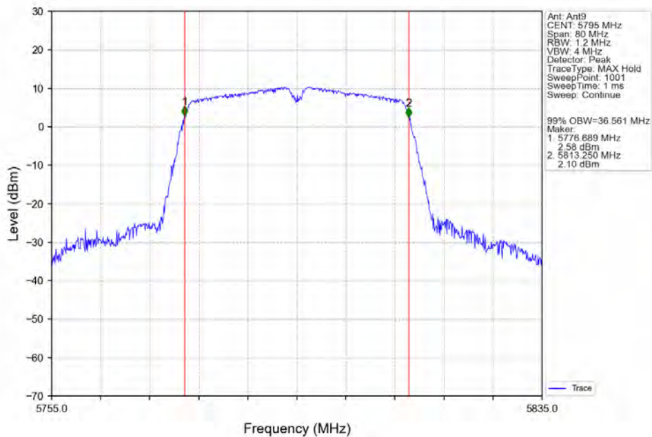
802.11ac(VHT40)_HCH_5795MHz_Ant9_NTNV
