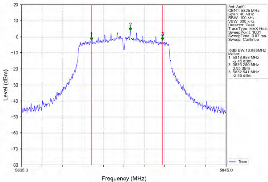
802.11n(HT20)_HCH_5825MHz_Ant9_NTNV
