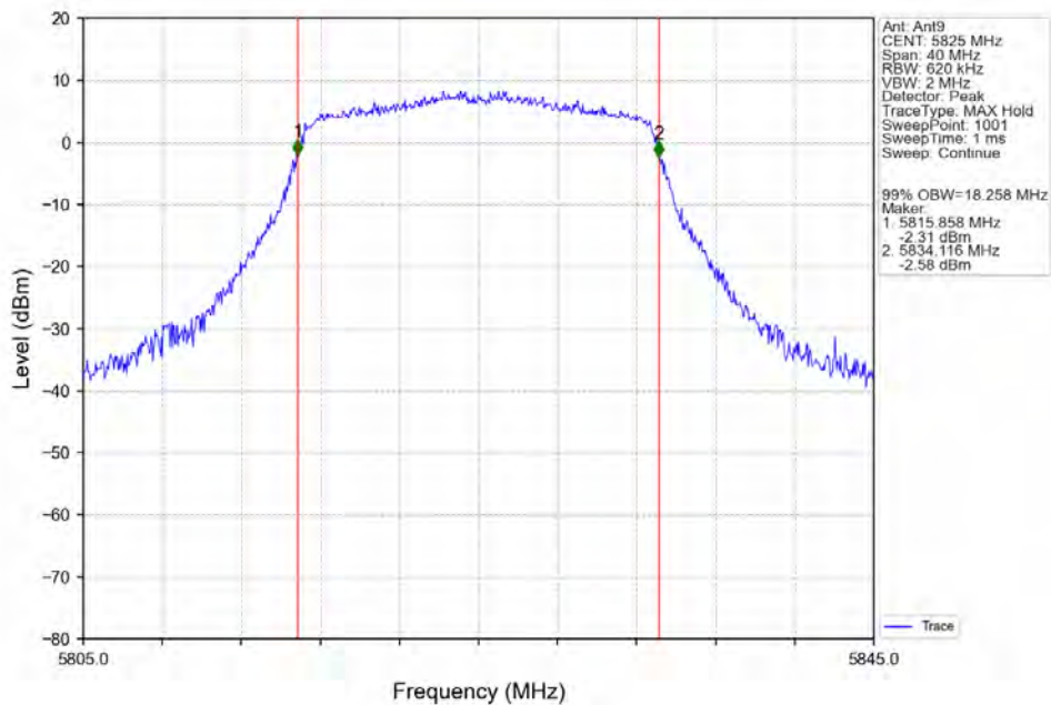
802.11n(HT20)_HCH_5825MHz_Ant9_NTNV
