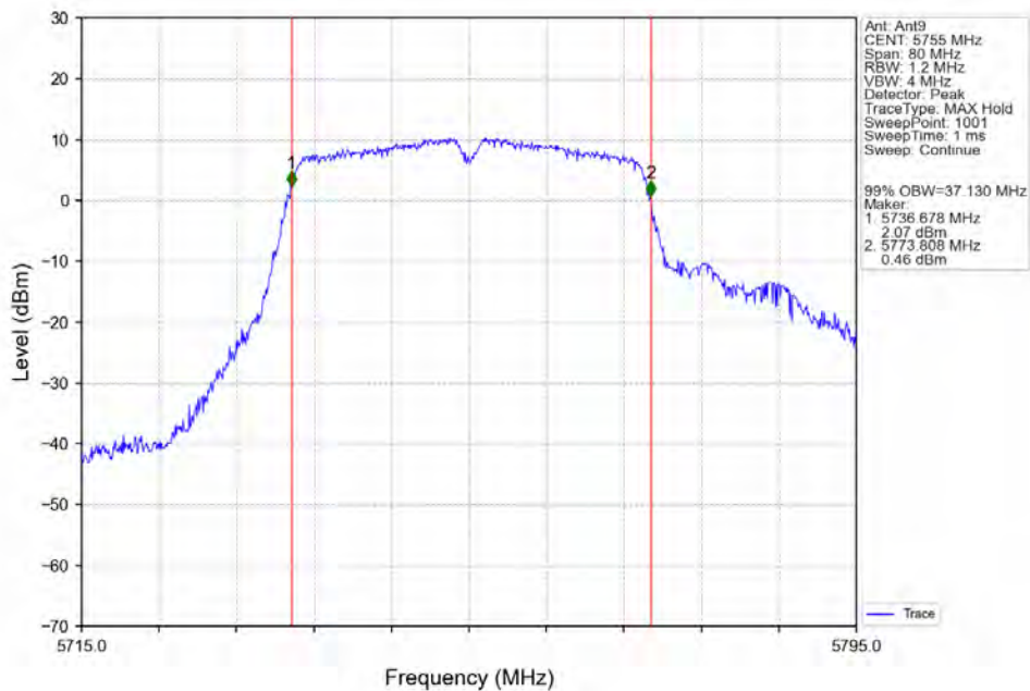
802.11n(HT40)_LCH_5755MHz_Ant9_NTNV
