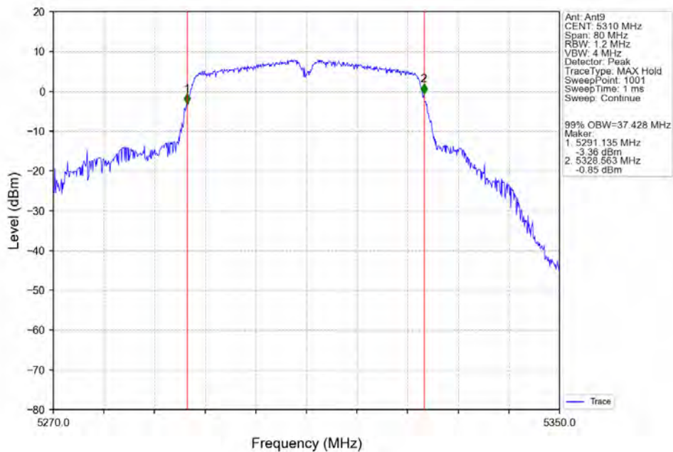
802.11n(HT40)_HCH_5310MHz_Ant9_NTNV
