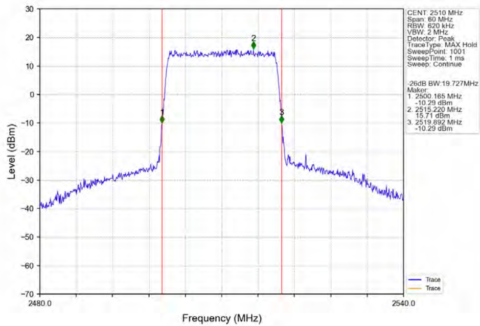
Band7_20MHz_256QAM_LCH_2510MHz_RB_100_0_NTN
