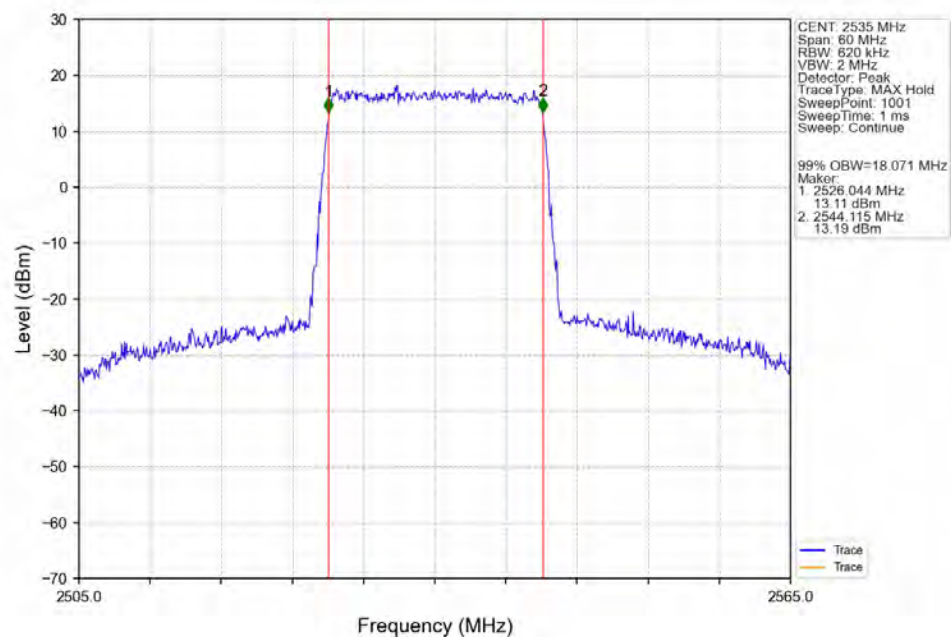
Band7_20MHz_64QAM_MCH_2535MHz_RB_100_0_NTNV
