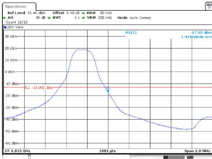
Band25-3MHz-QPSK-26675-1RB#14
