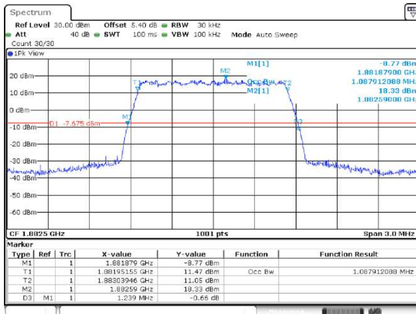
Band25-1.4MHz-QPSK-26365-6RB#0-1.088
