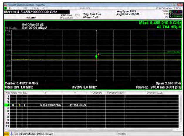
Band III 11ac40 CH102 AV
