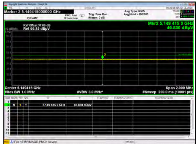
Band I 11ac40 CH38 AV
