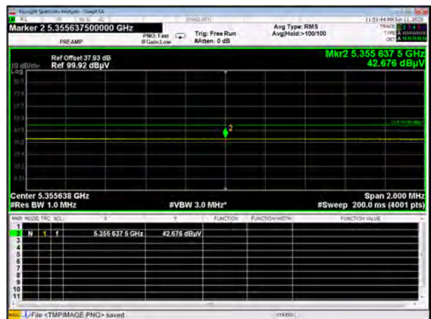
Band II 11ac20 CH64 AV
