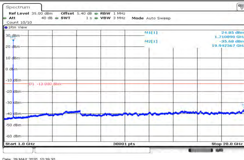
Band66-20MHz-QPSK-132072-1RB#0-Range2:1000~20000MHz
