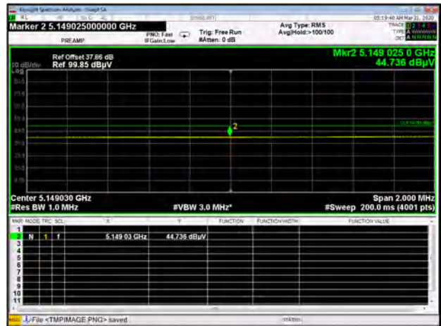
Band I 11n40 CH38 AV
