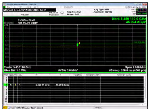
Band III 11ac80 CH106 AV
