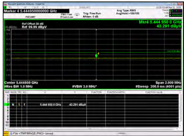
Band III 11n20 CH100 AV
