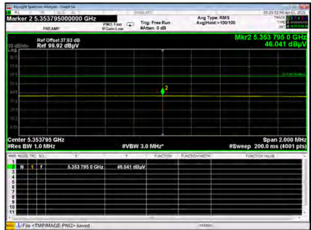
Band II 11a CH64 AV
