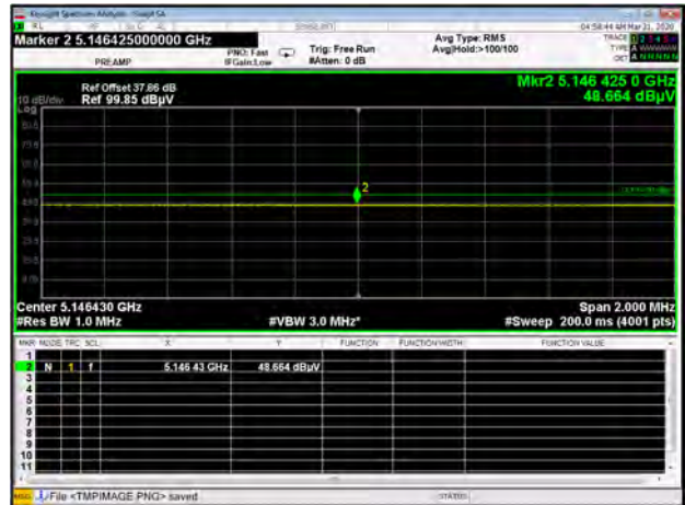
Band I 11ac80 CH42 AV
