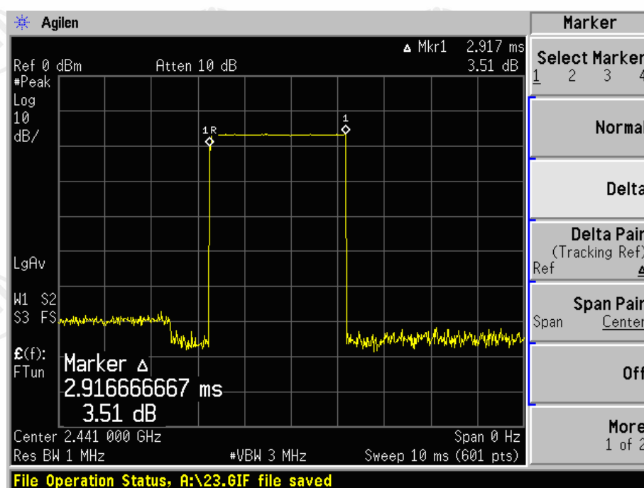
2441 MHz_DH5
