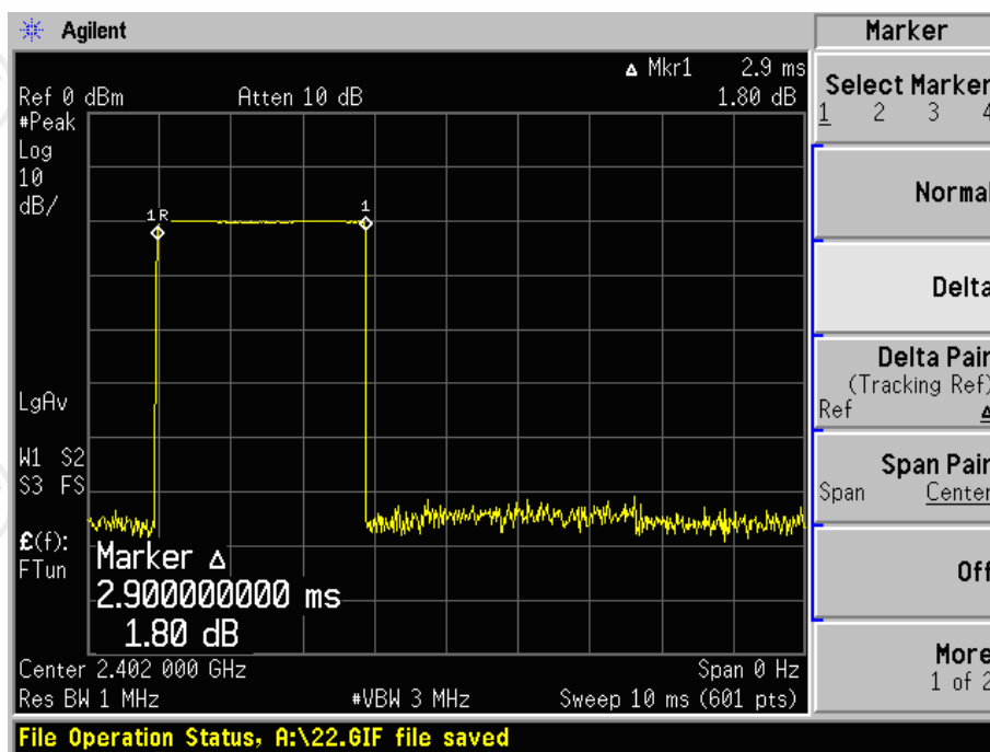
2402 MHz_DH5
