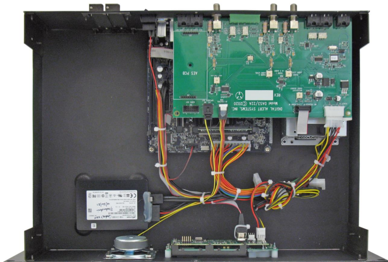
DASDEC-III Internal
