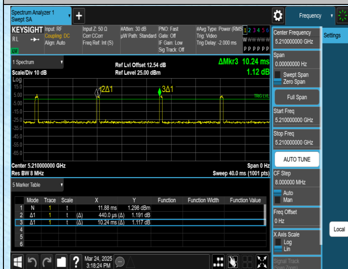
NTNV-11AC80MIMO-Ant1-5210
