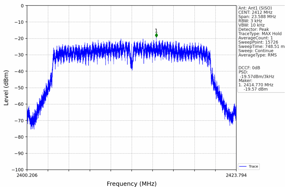
802.11n(HT20)_LCH_2412MHz_Ant1 (SISO)_NTNV
