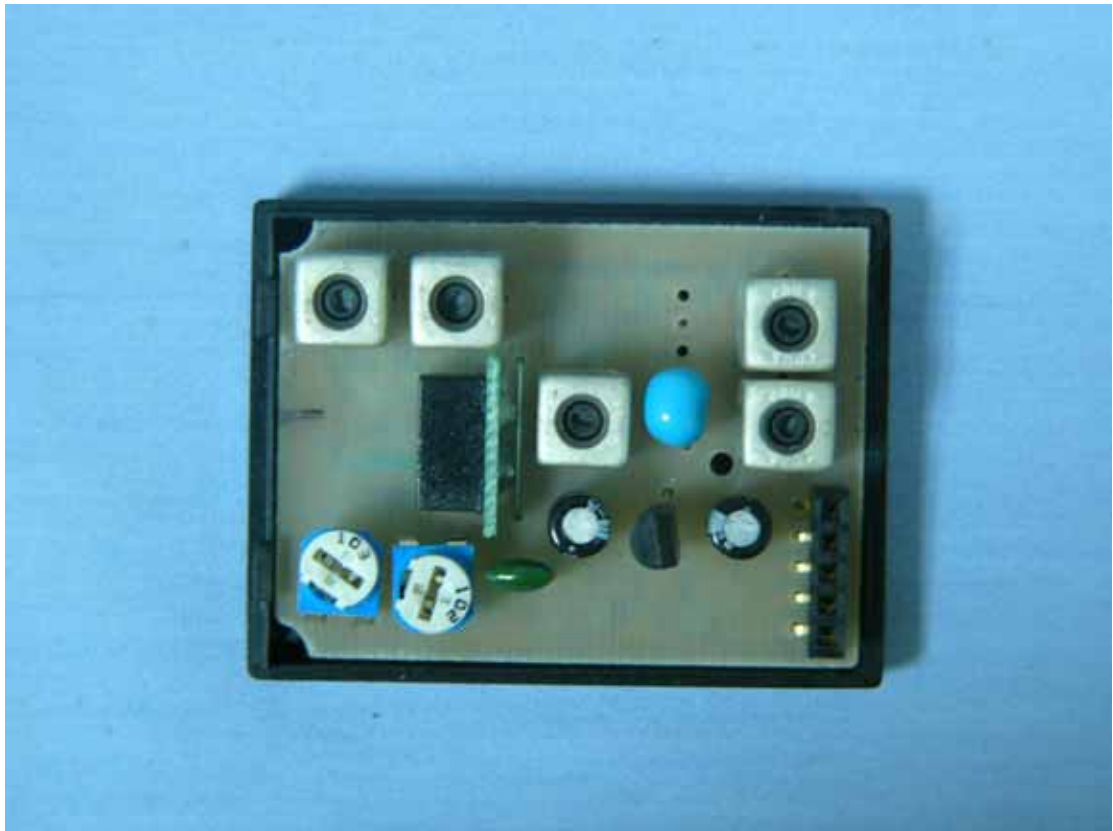
Transmitter module (72MHz)
