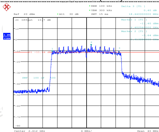
802.11ax(HT20)
