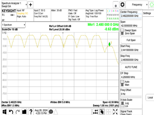
QPSK_SRD_2441-2480
