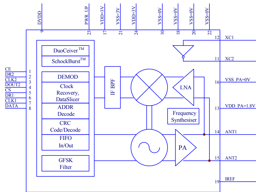
nRF2401
