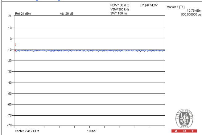
802.11n (HT20)
