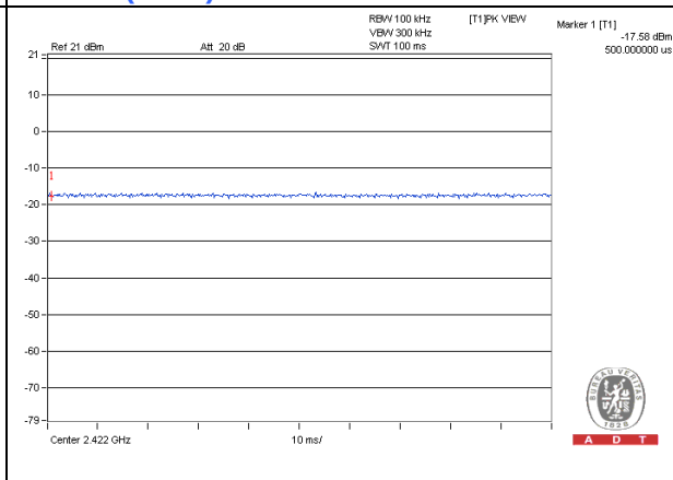
802.11n (HT40)
