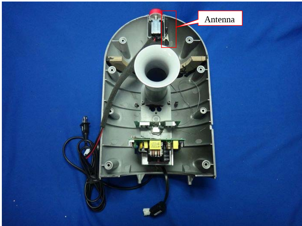
(18) EUT Photo
