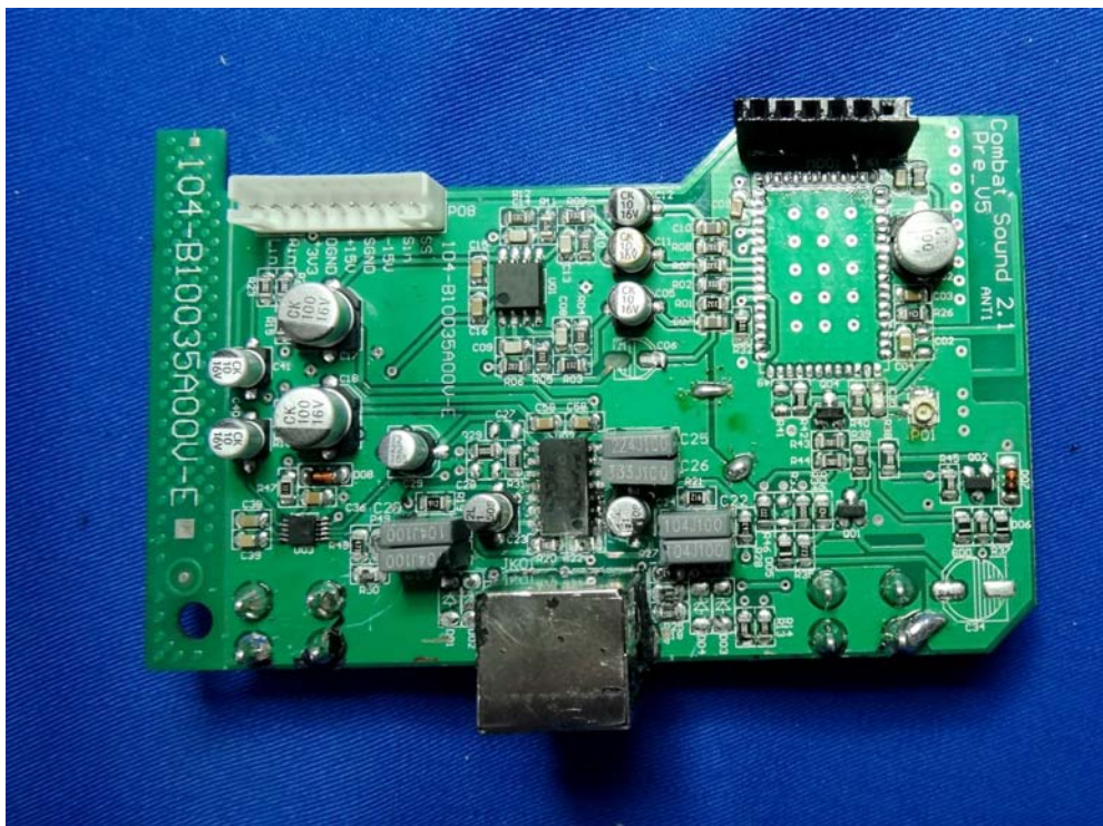
(24) EUT Photo
