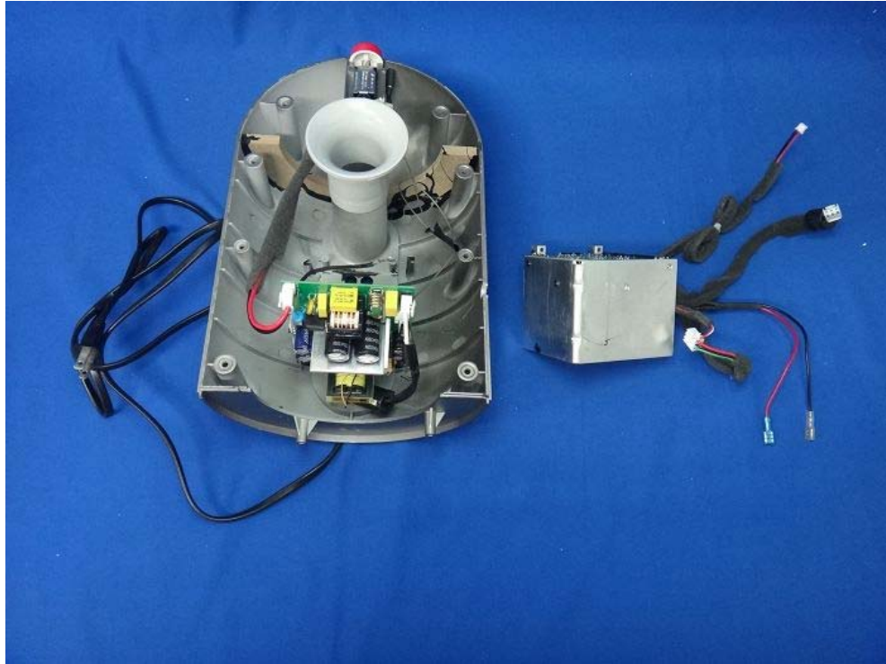
(13) EUT Photo
