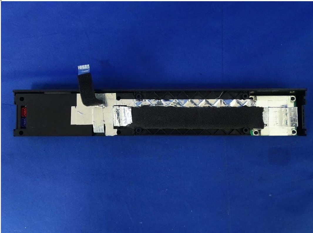
(14) EUT Photo
