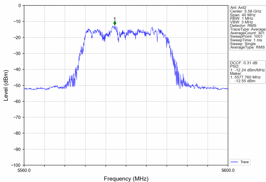
802.11n(HT20)_MCH_5580MHz_MIMO_NTNV
