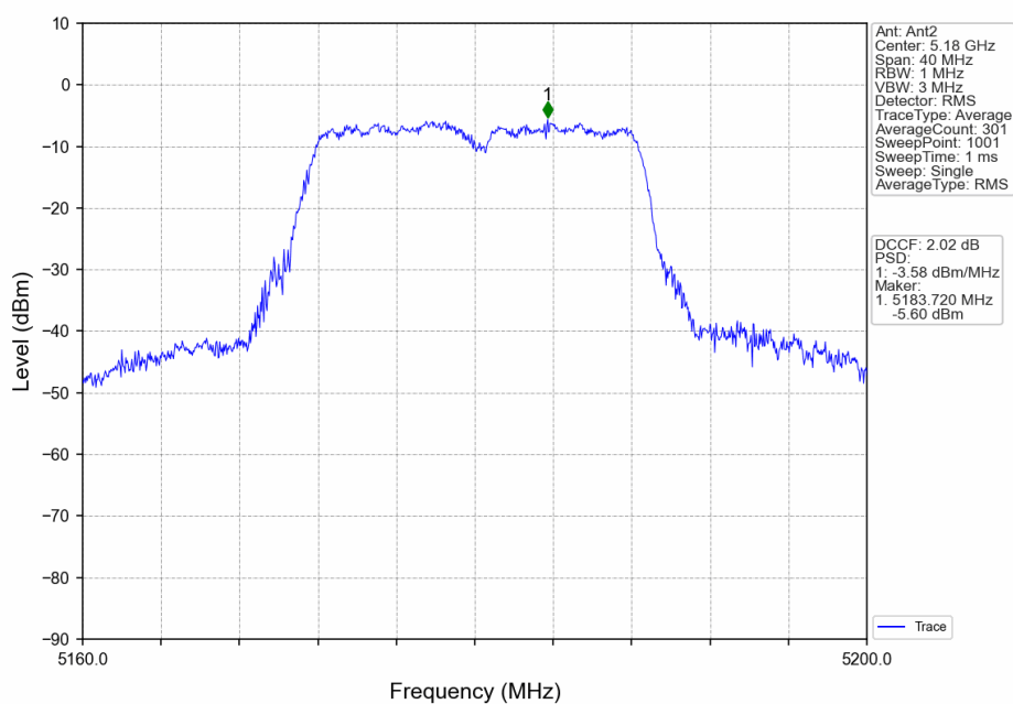
802.11n(HT20)_LCH_5180MHz_MIMO_NTNV
