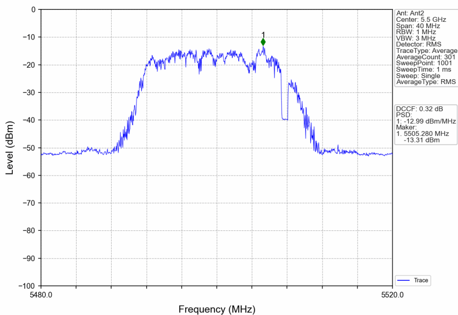
802.11n(HT20)_LCH_5500MHz_MIMO_NTNV
