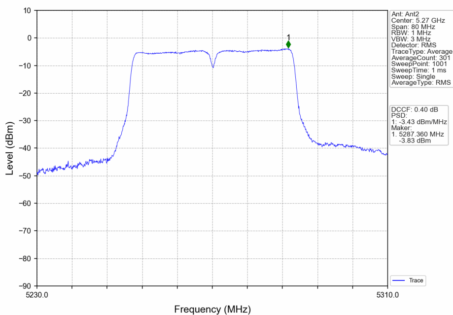
802.11n(HT40)_LCH_5270MHz_MIMO_NTNV
