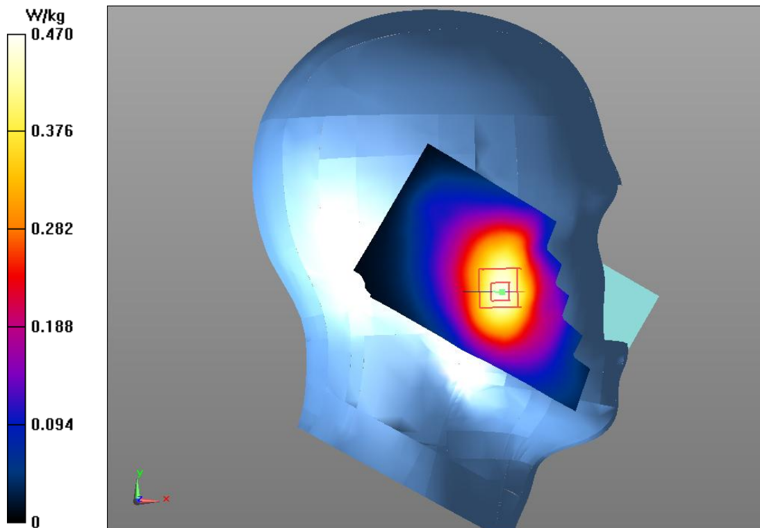
Fig.5 WCDMA 850 CH4182
