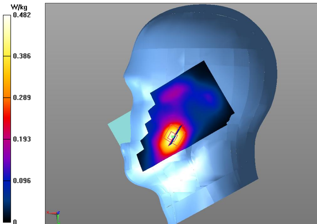
Fig.9 WCDMA1700 CH1413
