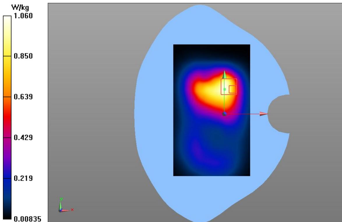
Fig.10 WCDMA1700 CH1513
