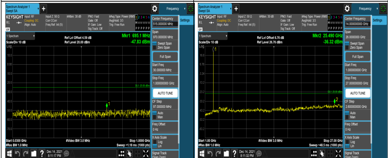
Band7-5MHz-QPSK-21425-1RB#0-Range1:30~100 0MHz
