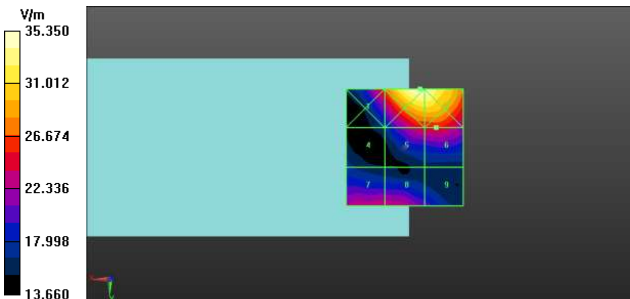
Fig A.10 HAC RF E-Field CDMA BC1
