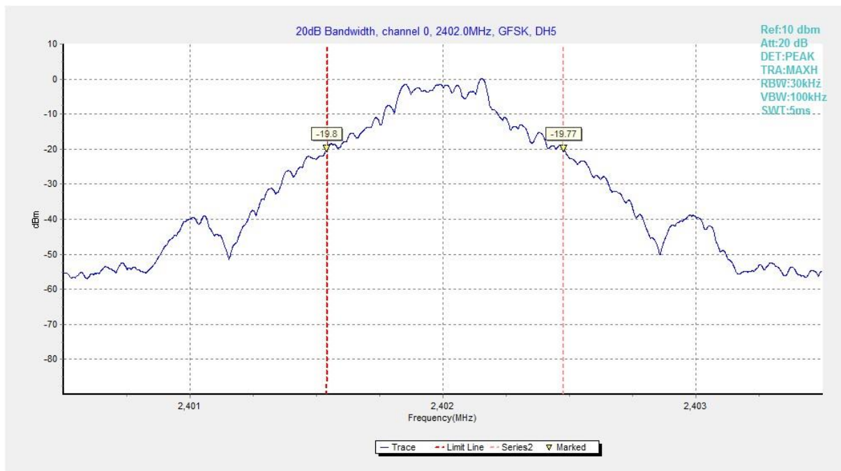
Fig. 78 20dB Bandwidth (GFSK, Ch 0)
