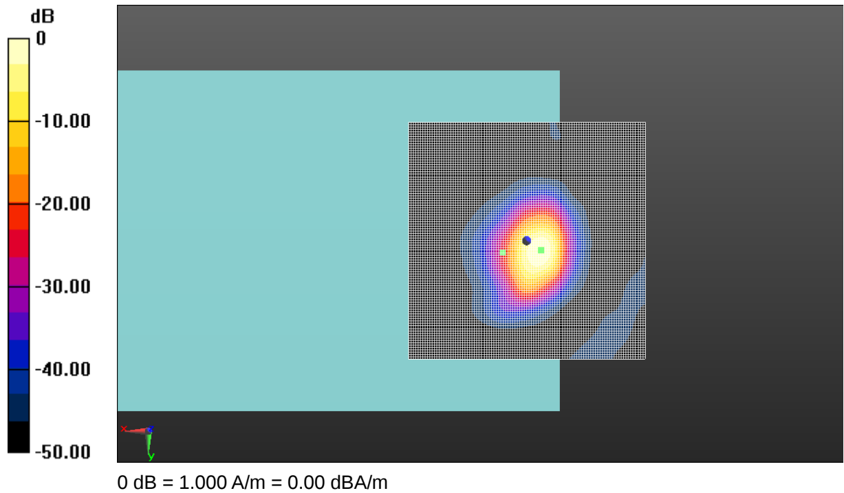
Fig A.6 T-Coil WCDMA B2-Z
