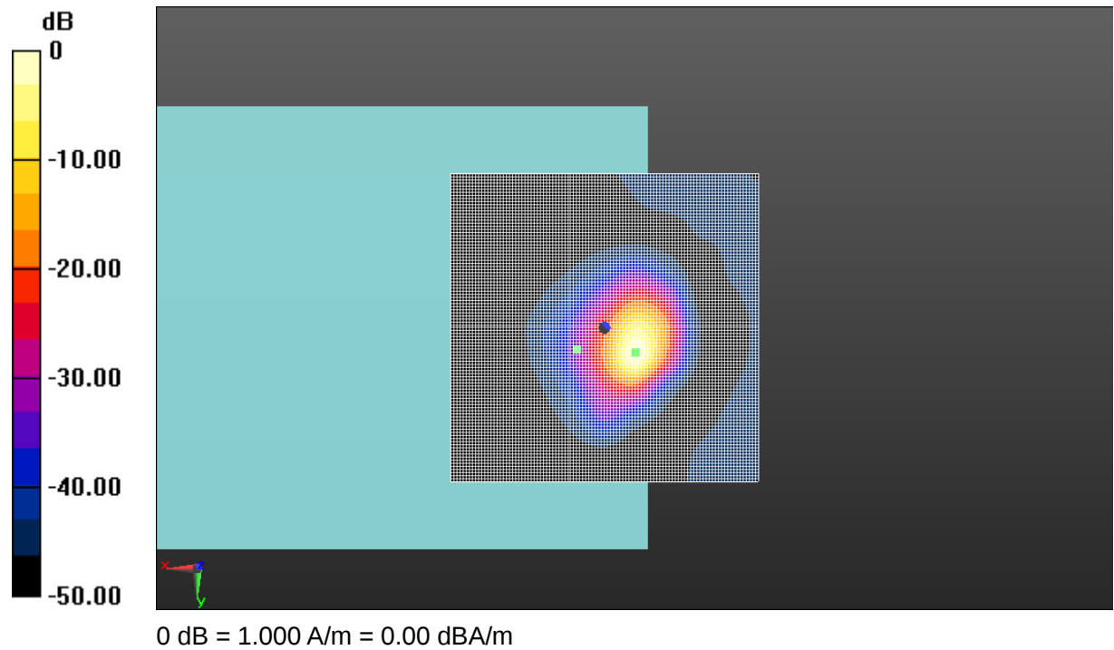
Fig A.15 T-Coil WCDMA B4-Z
