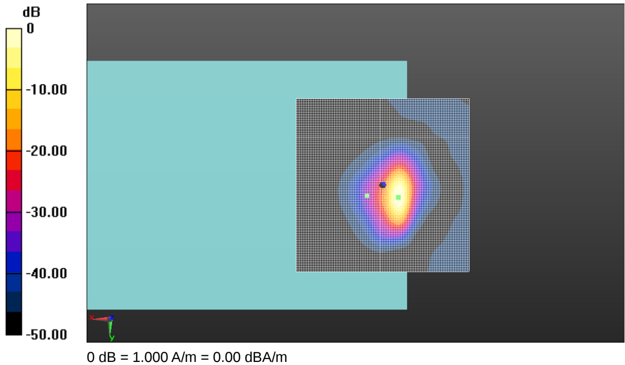
Fig A.16 T-Coil WCDMA B5-Z
