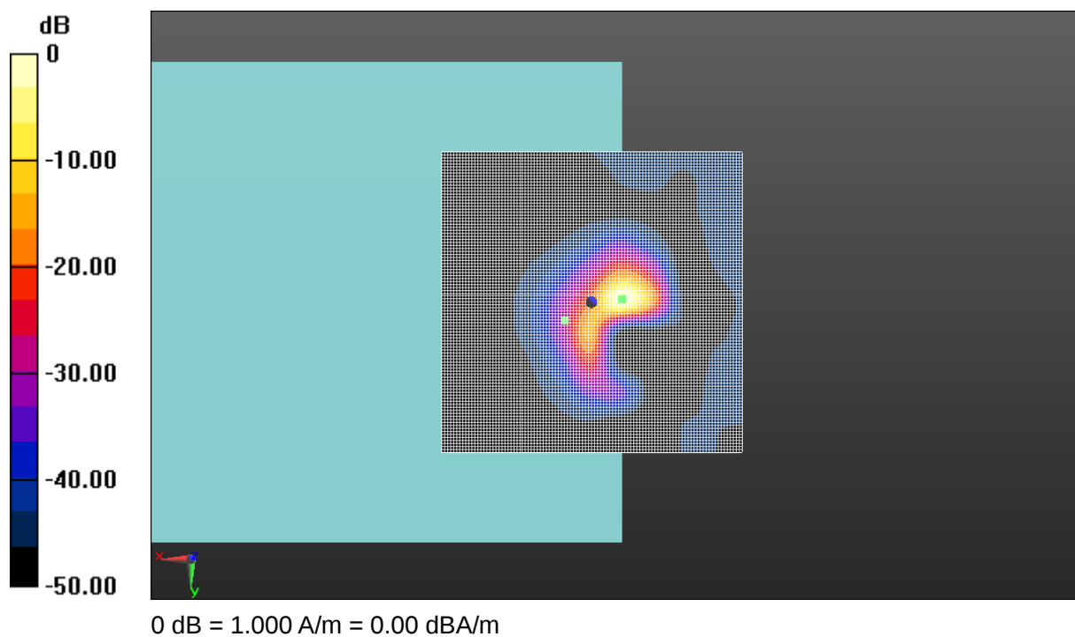
Fig A.11 T-Coil CDMA BC0-Z
