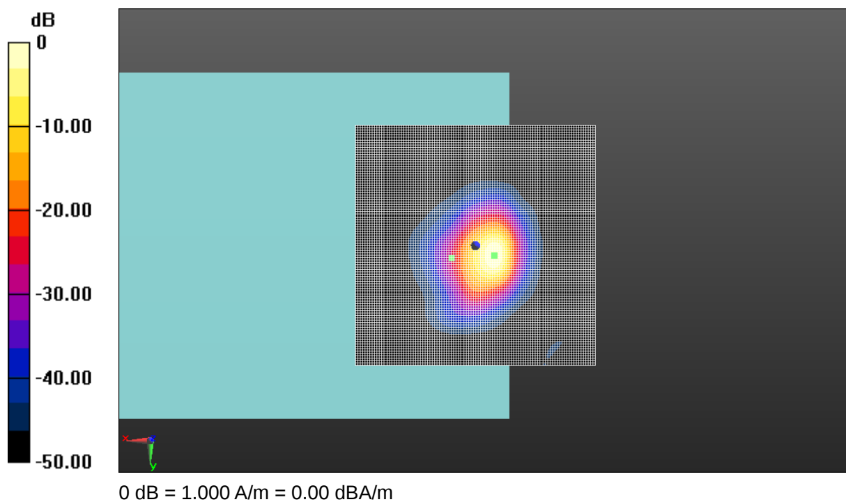
Fig A.8 T-Coil WCDMA B5-Z
