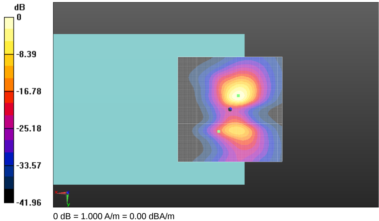
Fig A.7 T-Coil WCDMA B4-Y
