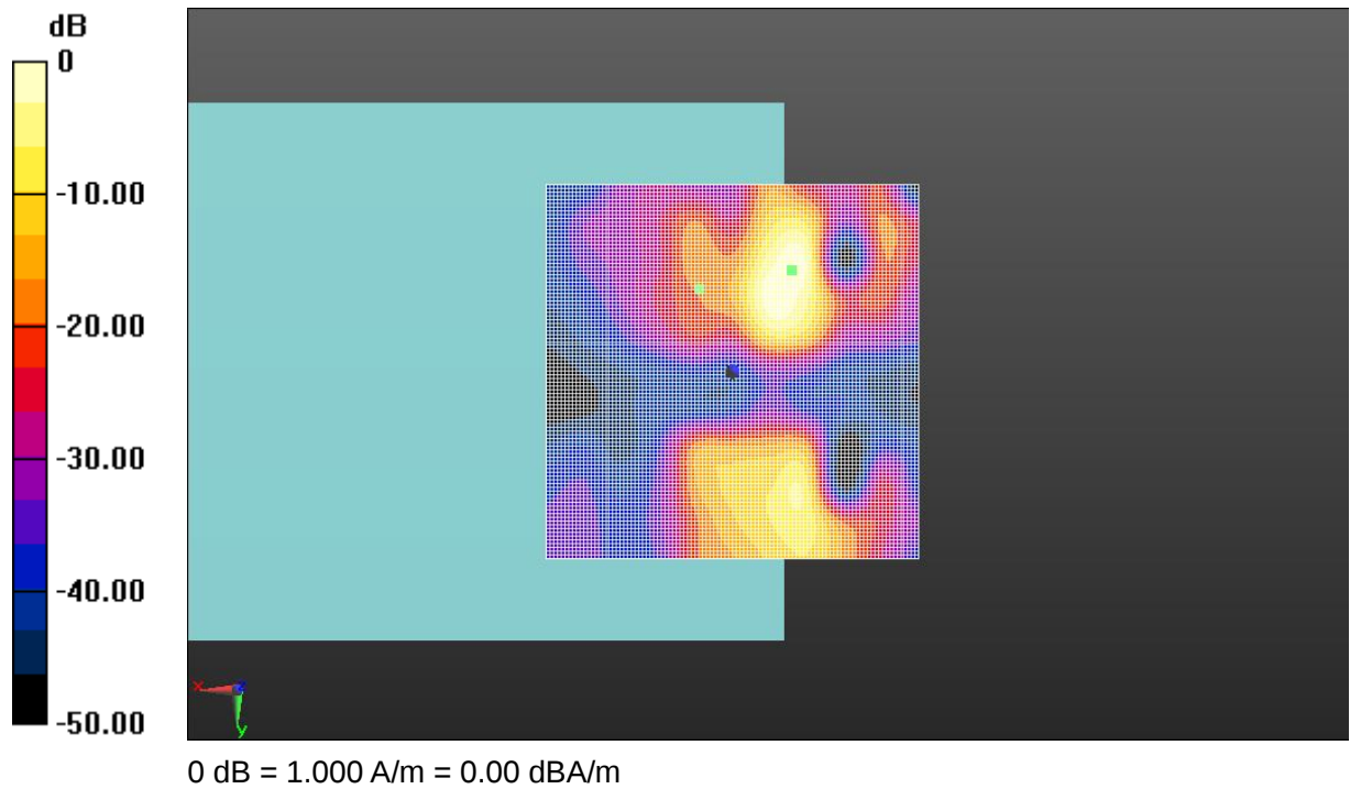
Fig A.9 T-Coil GSM 850-Y
