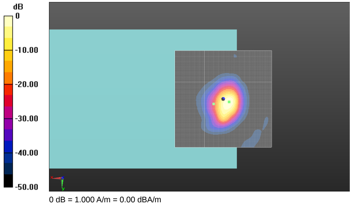
Fig A.7 T-Coil WCDMA B4-Z
