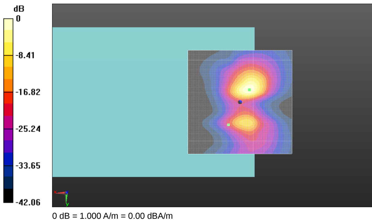
Fig A.6 T-Coil WCDMA B2-Y
