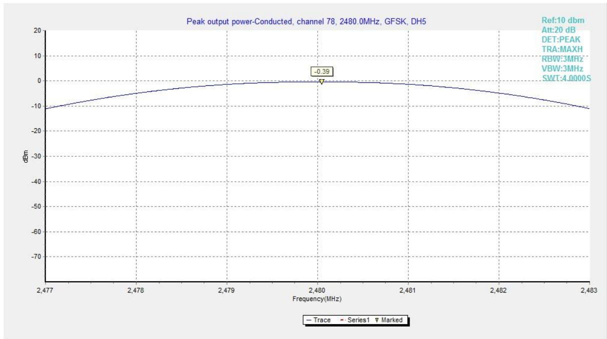
Fig. 3 RF output power (GFSK, Ch 78)
