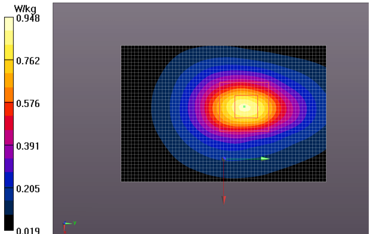
Fig.10 WCDMA1700
