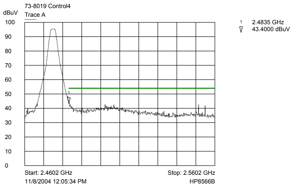
Trace A Upper Band Edge
