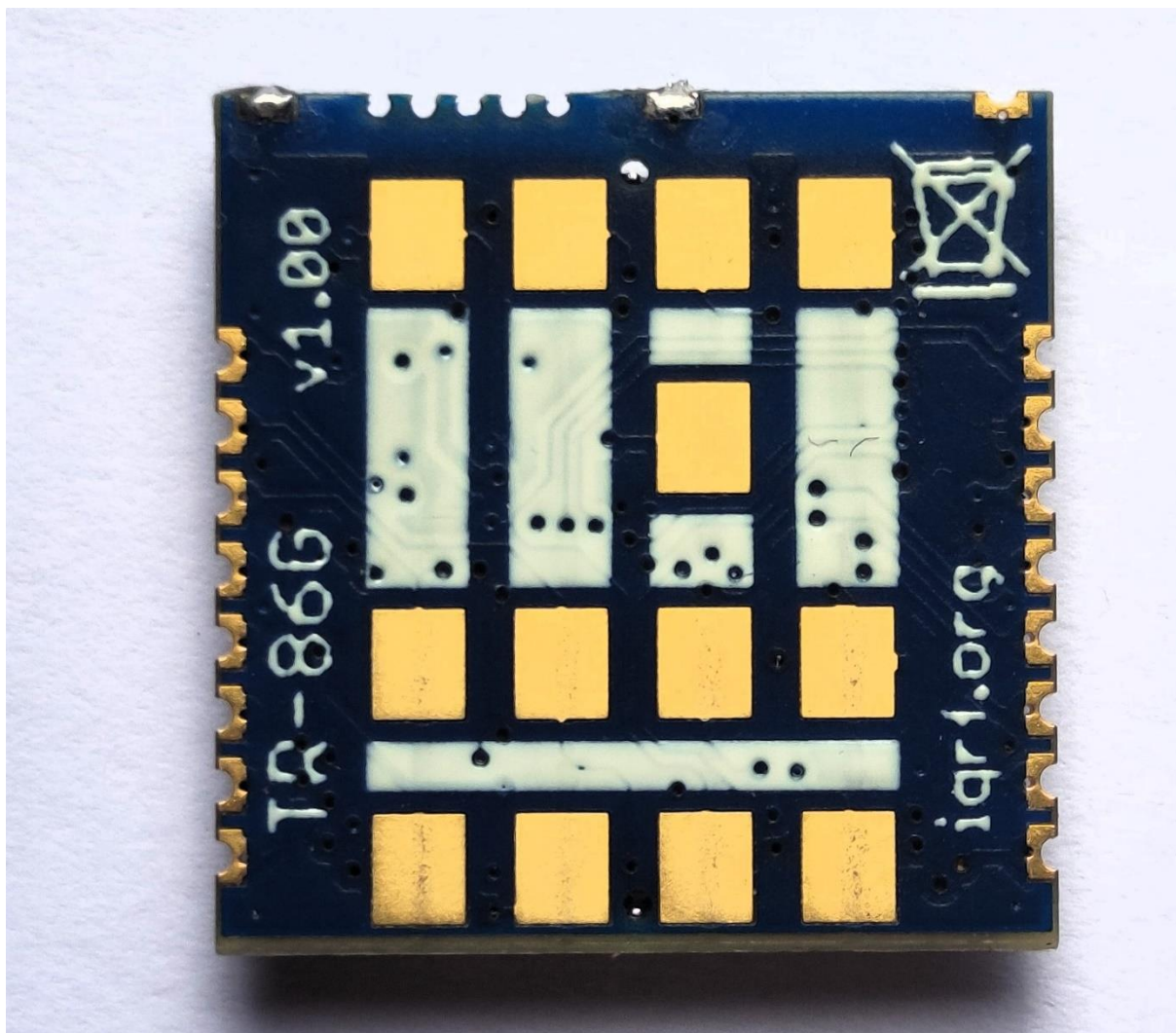
Figure 12: TR-86G, BOT
