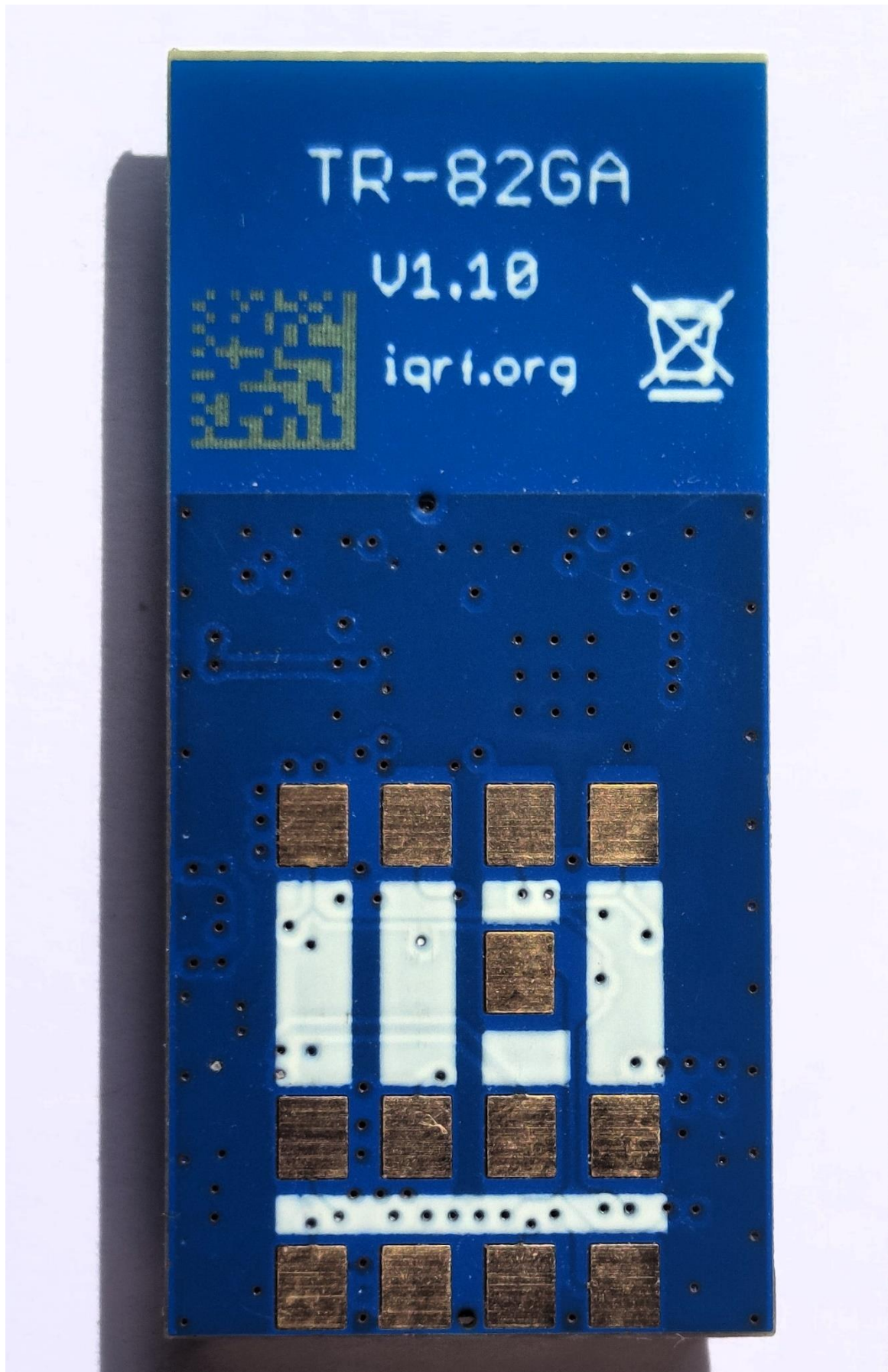
Figure 3: TR-82GA, BOT
