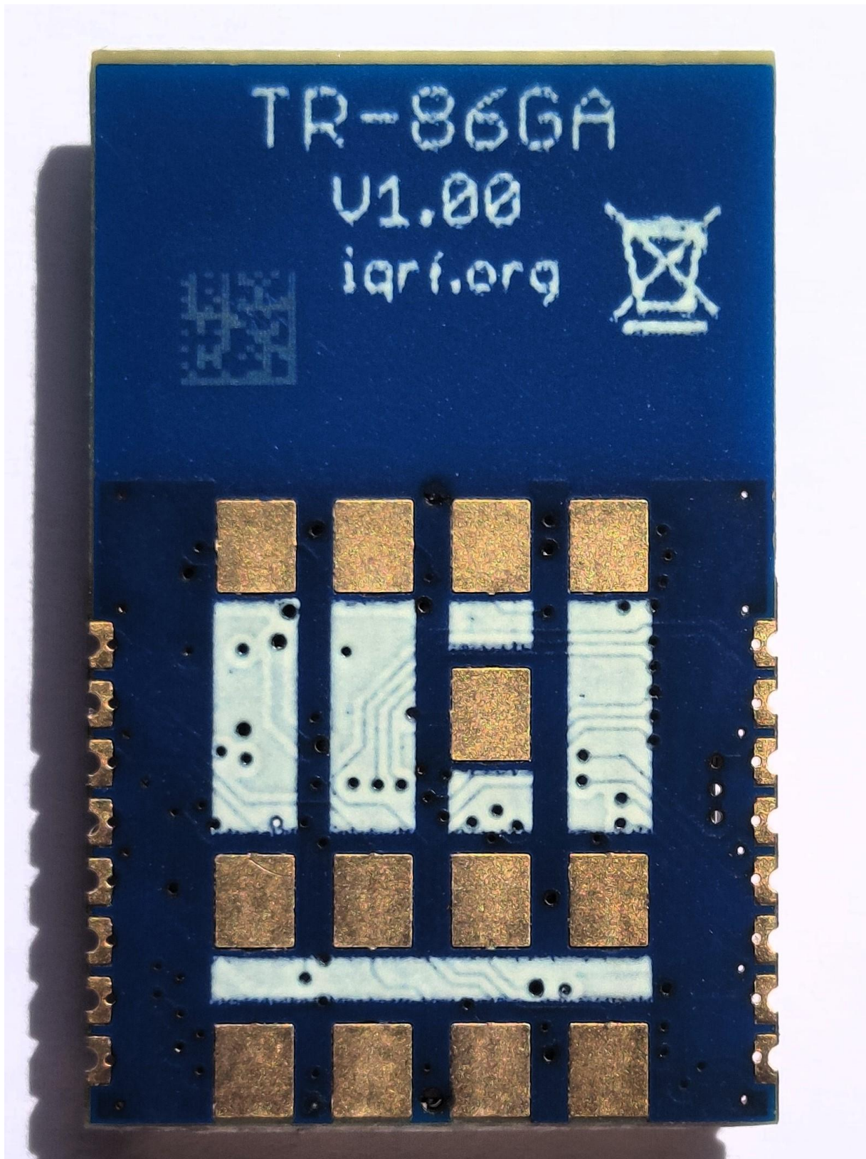
Figure 9: TR-86GA, BOT
