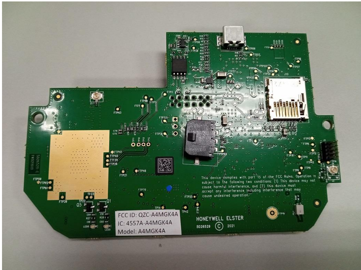
A4MGK4A PCBA Bottom Side
