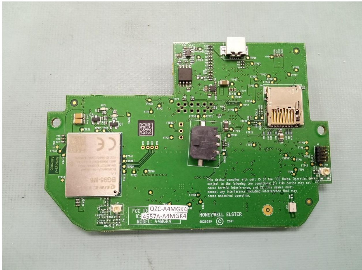
A4MGK4 PCBA Bottom Side
