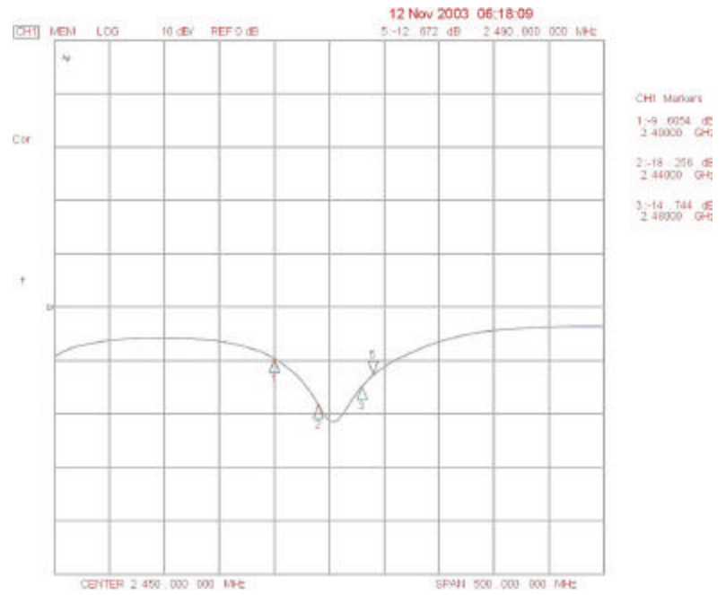
Fig 2. VSWR
