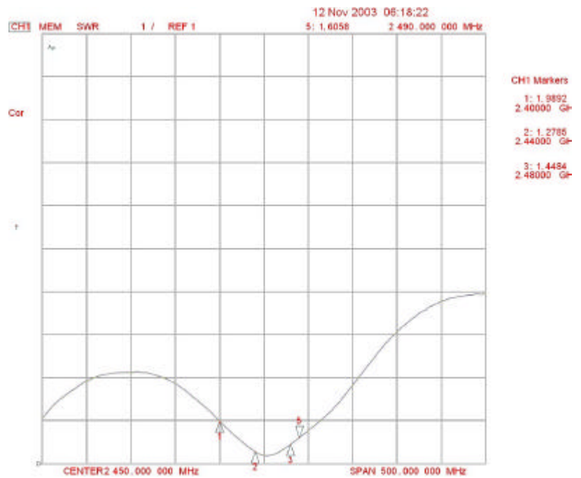
Fig 2. VSWR
