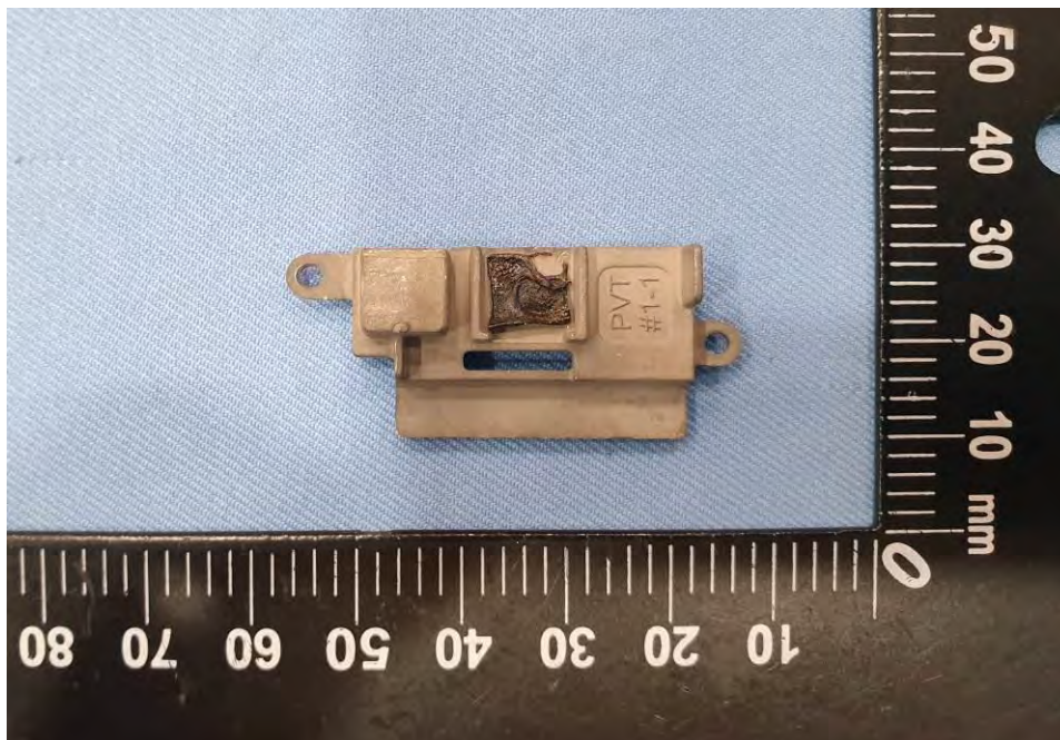
EUT Photo (30)
