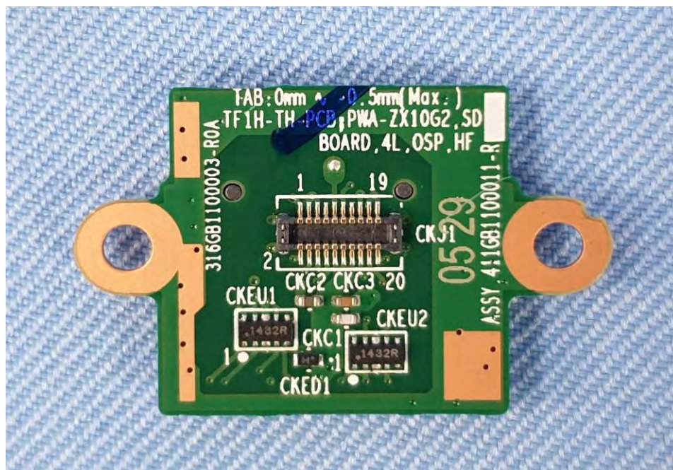
EUT Photo (36)
