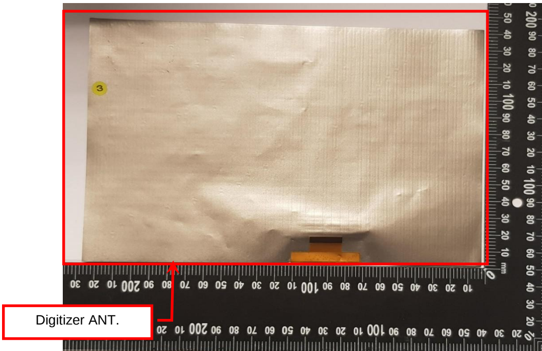
EUT Photo (4)
