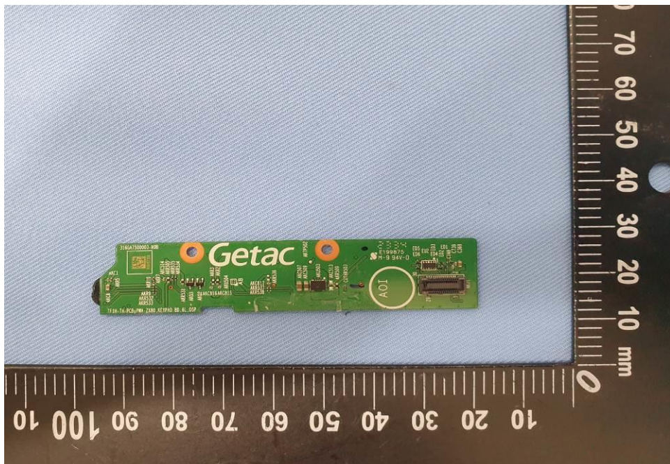
EUT Photo (88)
