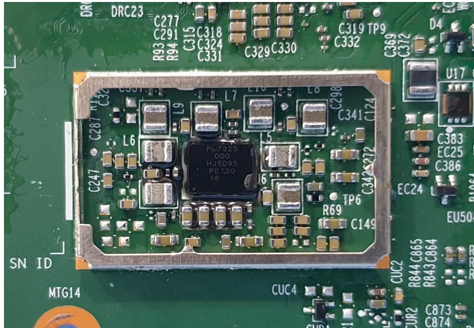
EUT Photo (54)
