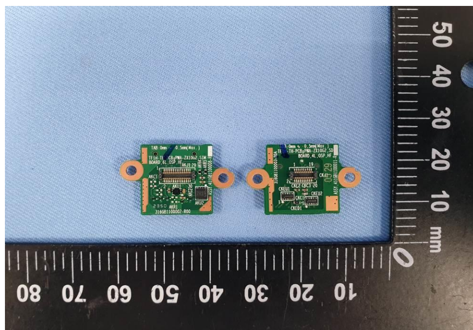
EUT Photo (36)
