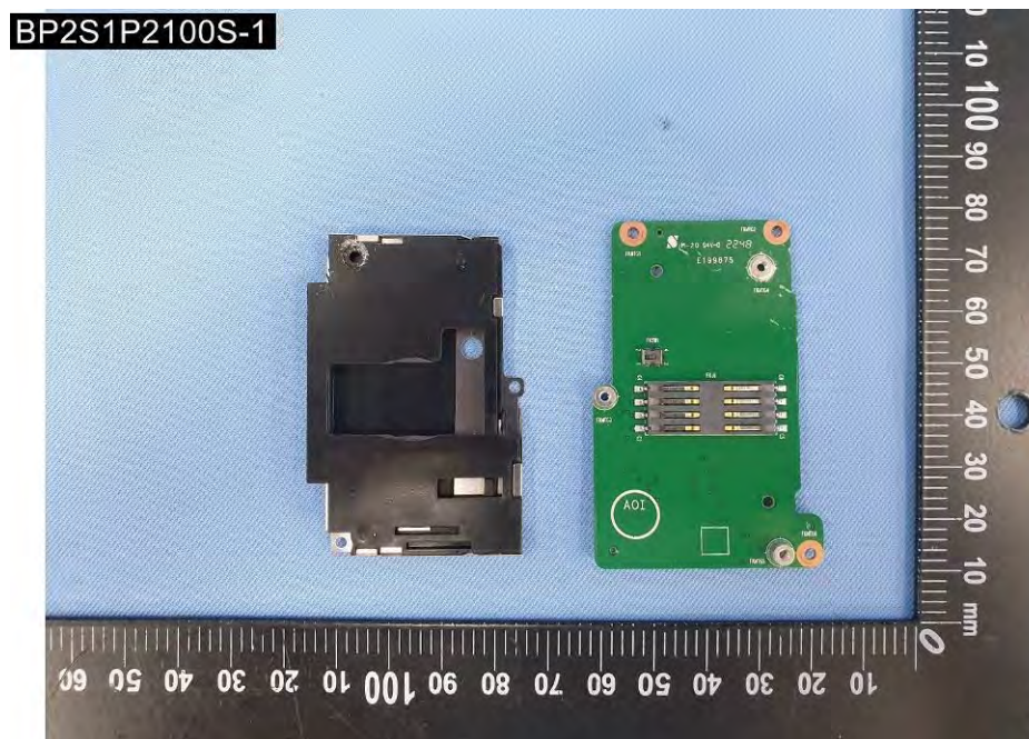
EUT Photo (142)
