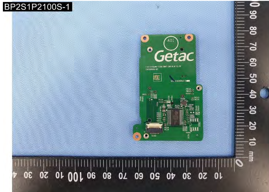
EUT Photo (144)
