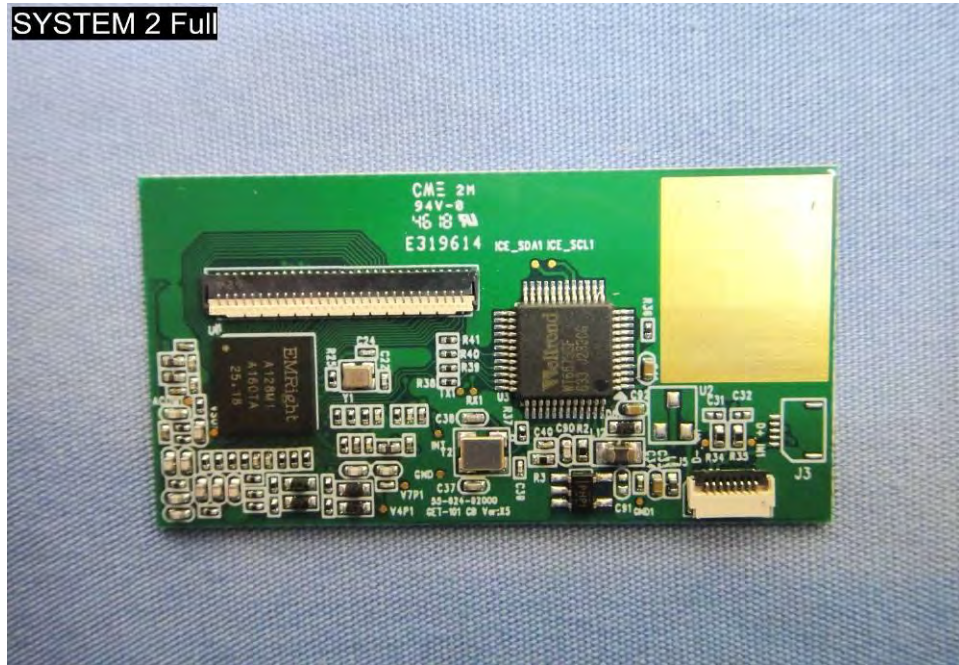
EUT Photo (122)
